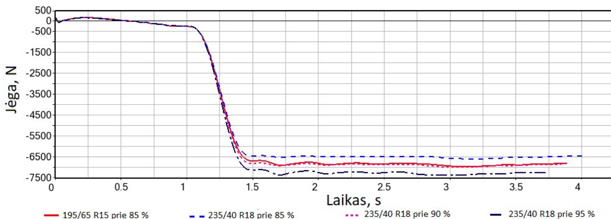
23 pav. Išilginės sukibimo jėgos, tenkančios priekiniams ratams stabdymo metu
