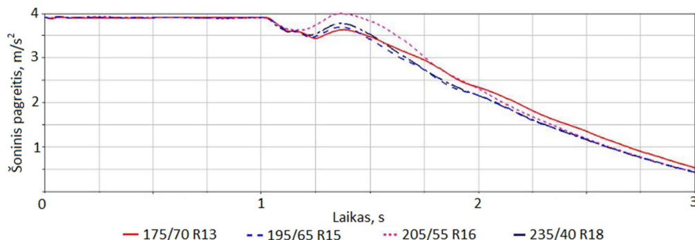
27 pav. Padangoms tenkantis šoninis pagreitis posūkio įveikimo metu
