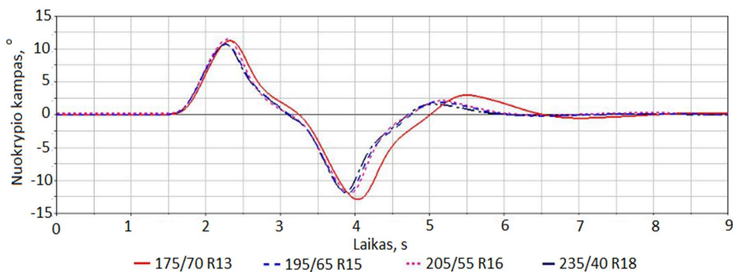
37 pav. Padangos nuokrypio (pasisukimo) kampas dvigubos juostos keitimo simuliacijos metu
