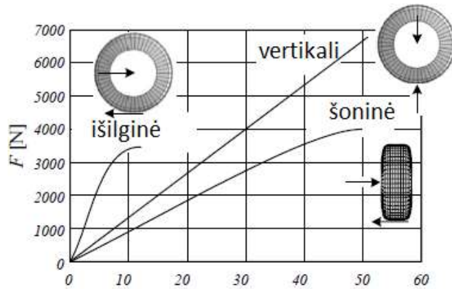
7 pav. Padangos deformacijos skirtingomis kryptimis (Jazar 2009)
