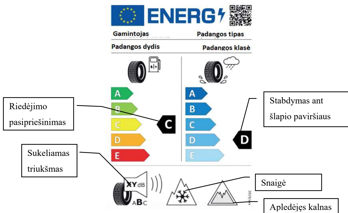
14 pav. Padangų etiketės ženklavimas pagal naujausią (ES) 2020/740 reglamentą
