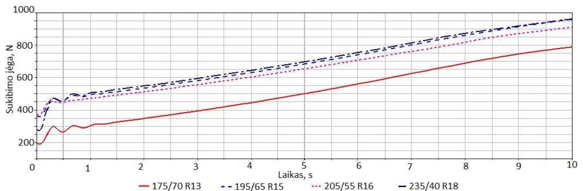
41 pav. Skersinio sukibimo jėga, tenkanti priekinei kairiajai padangai posūkio metu, esant pastoviam spinduliui
