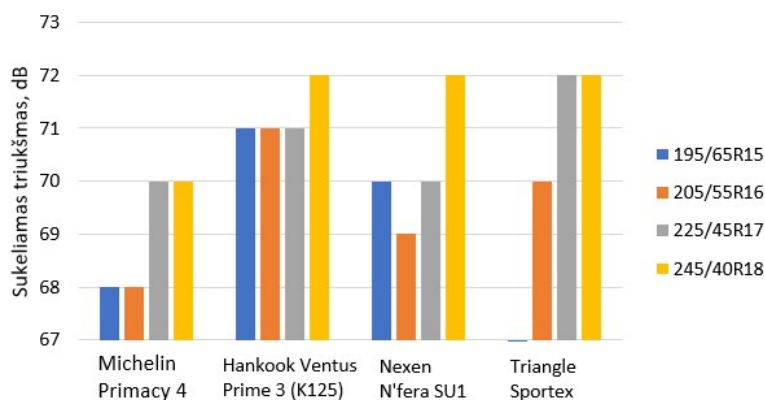
16 pav. Padangų sukeliama triukšmas pagal padangų matmenis
