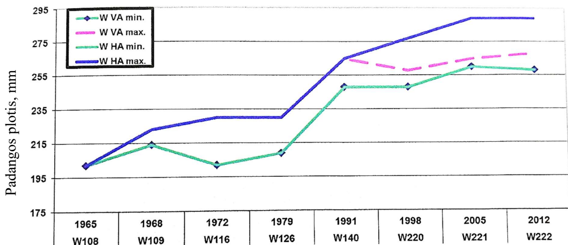
5 pav. S klasės Mercedes-Benz gamintojo rekomenduojamų padangų pločiai pagal modelį ir metus (Leister 2018)
