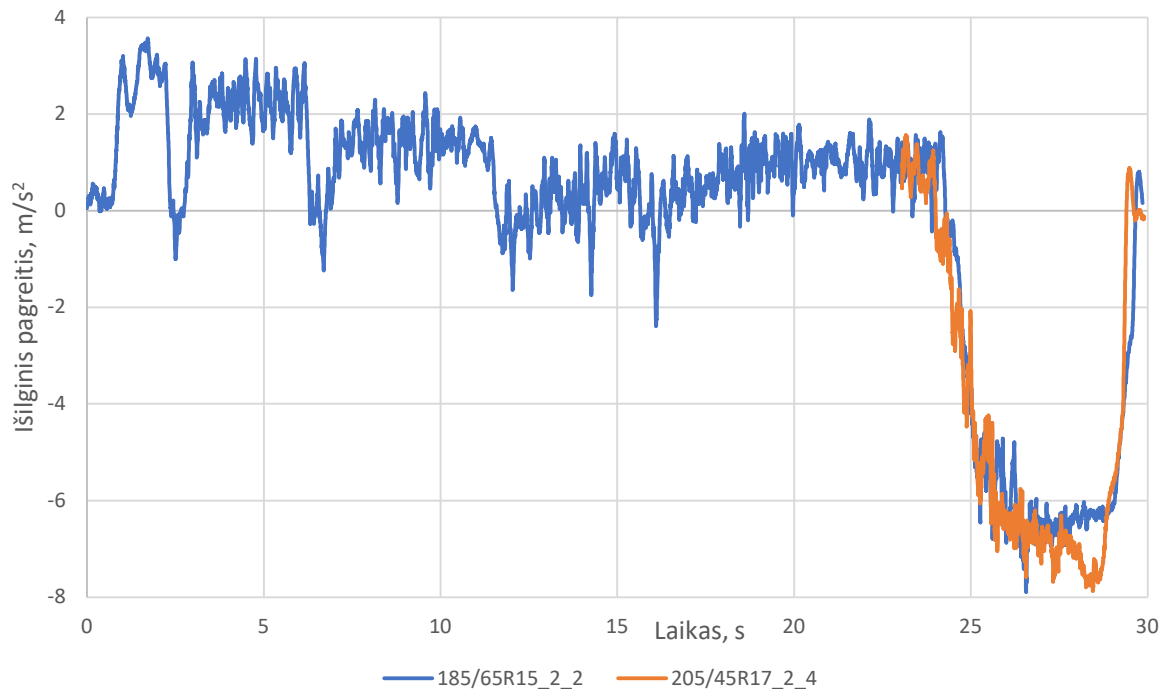
48 pav. Išilginio pagreičio pagal laiką grafikas stabdymo eksperimentinių tyrimo metu, kai skirtumas tarp stabdymo laiko yra antras pagal mažumą
