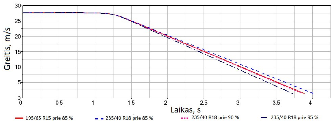
25 pav. Padangos stabdymo greitis stabdymo metu
