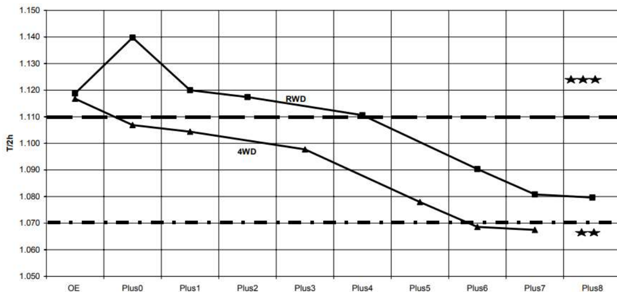
12 pav. Statinio stabilumo faktoriaus tyrimas, atliekant tyrimą su skirtingo dydžio ratlankiais ir padangomis (Daws 2005)
