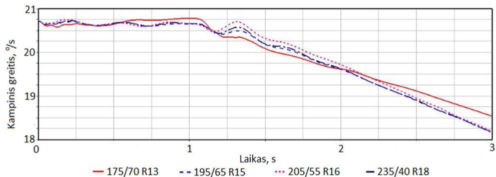
32 pav. Kampinis greitis stabdymo posūkyje metu
