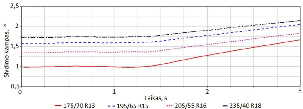
33 pav. Padangoms tenkantis slydimo kampas stabdymo posūkyje metu
