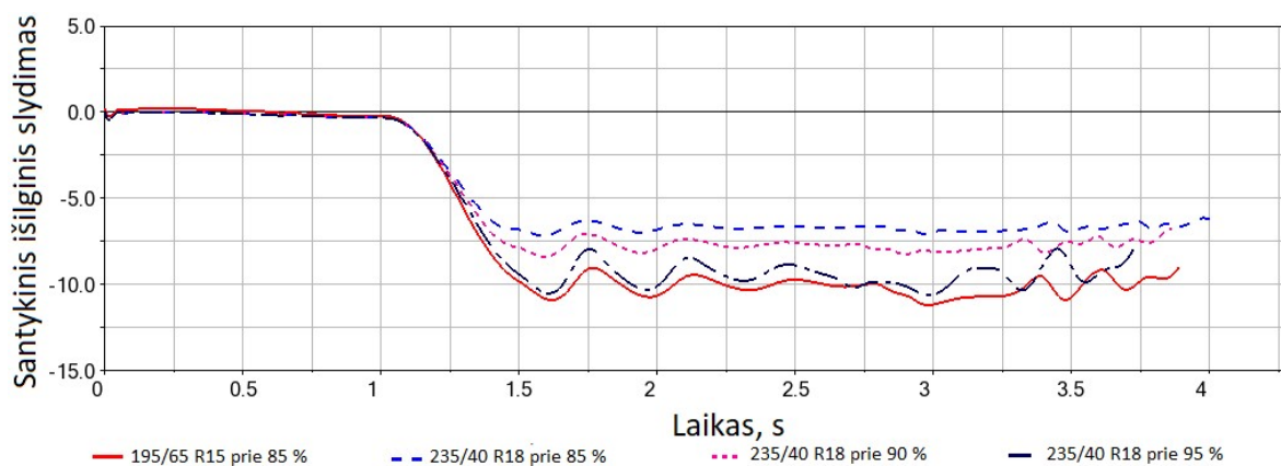
22 pav. Padangos santykinis slydimas, tenkantis priekiniam kairiajam ratui stabdymo metu neužblokuotiems ratams
