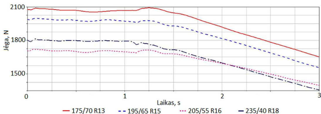
34 pav. Priekinei kairei padangai tenkanti skersinė sukibimo jėga stabdymo posūkyje metu
