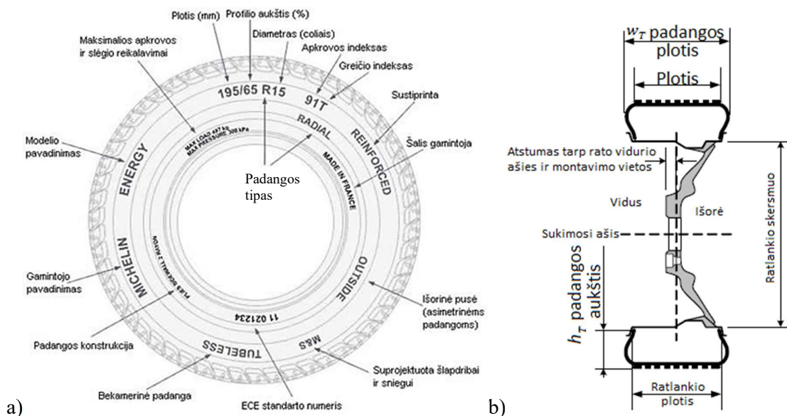
2 pav. Rato matmenys: a) Padangos charakteristikas vaizduojanti informacija ant padangos šono ( automanas.autobilis.lt ); b) ratlankio skerspjūvis su pagrindiniais matmenimis (Jazar 2009)
