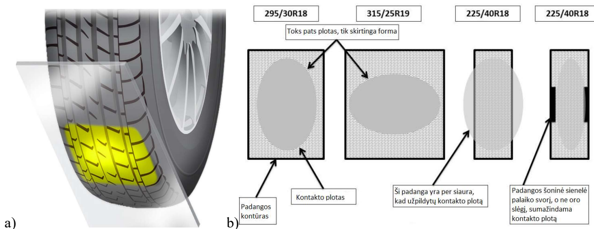
4 pav. a) Padangos kontakto plotas su kelio paviršiu ( 17to40.co.uk/the-tire... ); b) padangos kontakto priklausomybė nuo padangos geometrijos ( 6speedonline.com/forums/996-turbo... );
