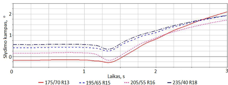
29 pav. Padangoms tenkantis slydimo kampas posūkio įveikimo metu
