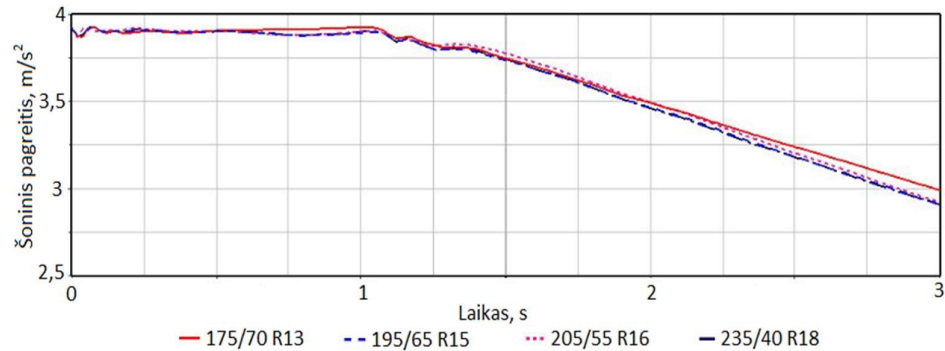
31 pav. Šoninis pagreitis stabdymo posūkyje metu
