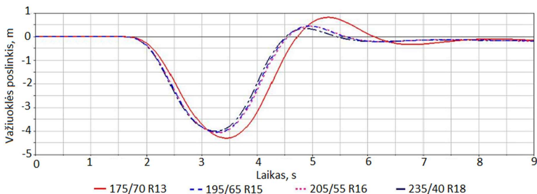
35 pav. Vaziuklės poslinkiai dvigubos juostos keitimo simuliacijos metu
