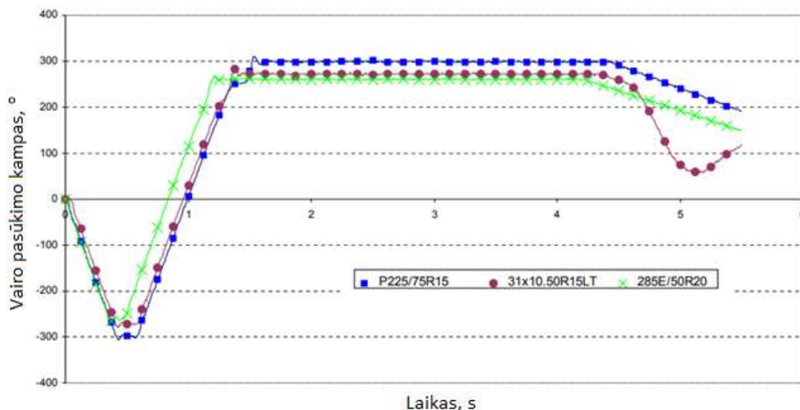
13 pav. Ratų pasūkimo kampas per laiką. Tyrimas atliekamas stovinčiam automobiliui (Daws 2005)
