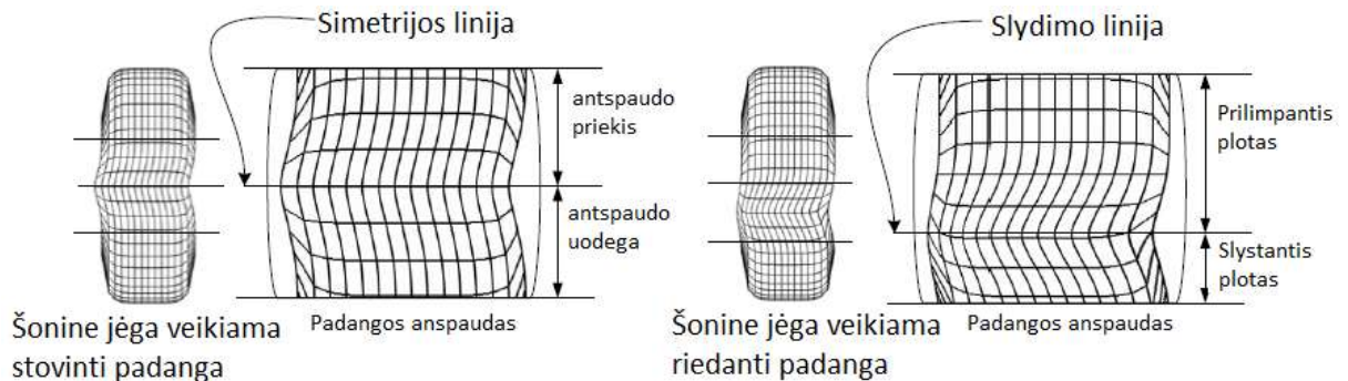
8 pav. Padangos antspaudas, kuomet padangą veikia šoninė jėga stovint ir riedant (Jazar 2009)
