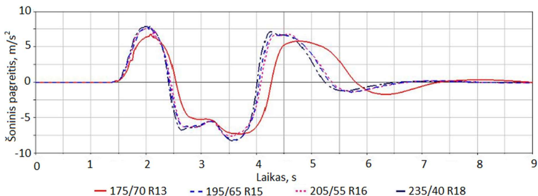
36 pav. Padangoms tenkantis šoninis pagreitis dvigubos juostos keitimo simuliacijos metu
