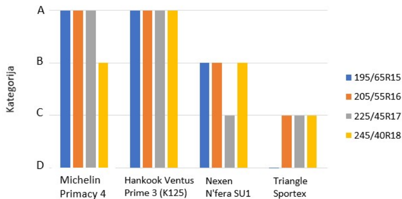
15 pav. Stabdymo ant šlapios dangos indeksai pagal padangų matmenis
