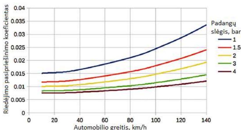
11 pav. Padangos riedėjimo pasipriešinimo priklausomybė nuo slėgio padangose ir važiavimo greičio (Mohanta, 2021)
