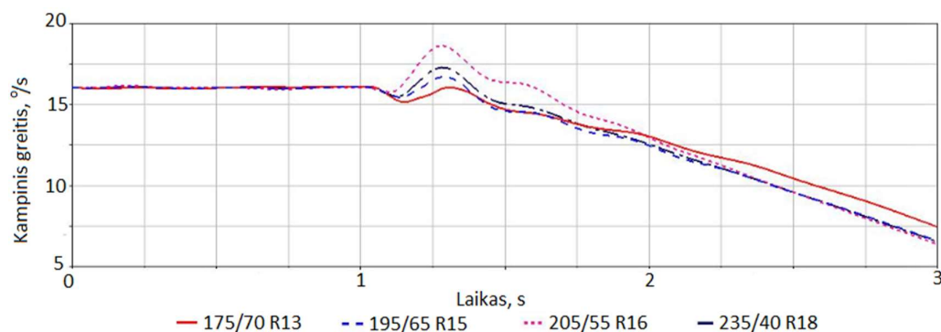
28 pav. Padangoms tenkantis kampinis greitis posūkio įveikimo metu
