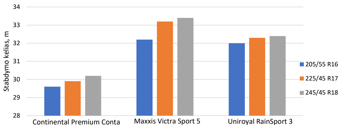
19 pav. Auto Bild ekspertų atliktų testų rezultatai stabdant 80–0 km/h ant šlapios dangos.
