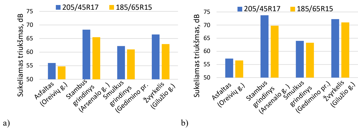
51 pav. Padangų sukeliamas triukšmas dB, pagal skirtingas kelio dangas: a) prie 30 km/h greičio, b) prie 50 km/h greičio
