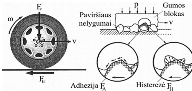
10 pav. Adhezijos ir histerezės jėgų veikiamos padangos deformacijos (Ružinskas 2018)
