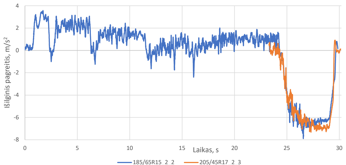
46 pav. Išilginio pagreičio pagal laiką grafikas stabdymo eksperimentinių tyrimo metu, kai skirtumas tarp stabdymo kelio yra mažiausias
