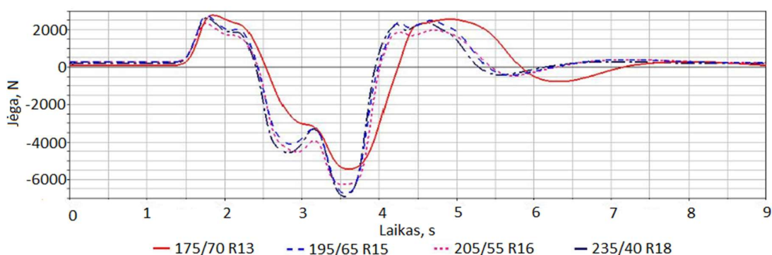
39 pav. Priekinę kairiąją padangą veikiančios šoninės jėgos dydis dvigubos juostos keitimo simuliacijos metu
