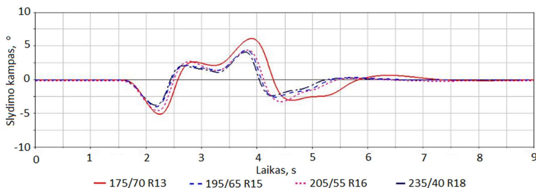
38 pav. Padangoms tenkančios skersridės kampas dvigubos juostos keitimo simuliacijos metu
