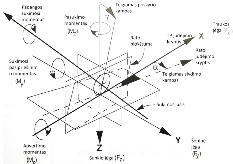
6 pav. Jėgos ir momentai veikiantys ratą (Gillespie 1992)
