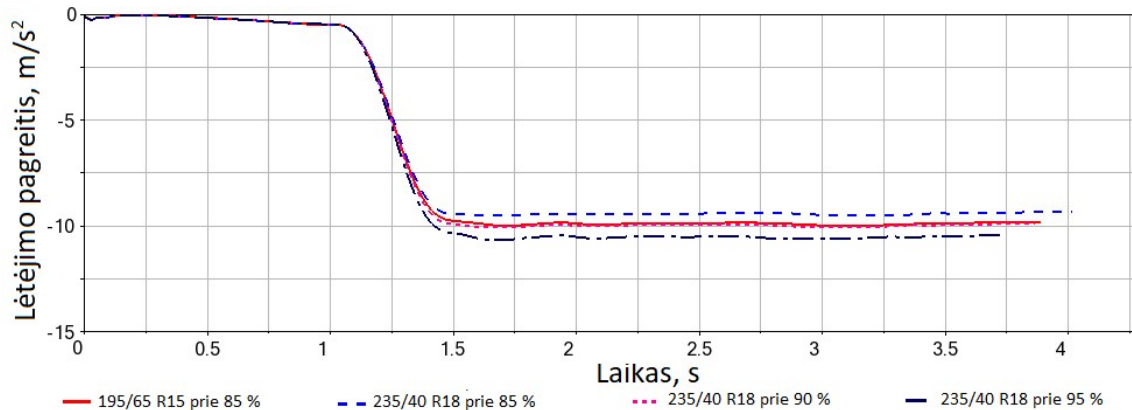
26 pav. Automobilio lėtėjimo pagreitis
