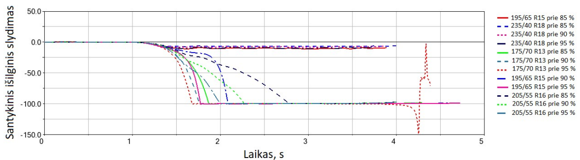
21 pav. Padangos santykinis išilginis slydimas, tenkantis priekiniam kairiajam ratui stabdymo metu
