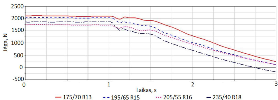
30 pav. Priekinei kairei padangai tenkanti šoninė sukibimo jėga
