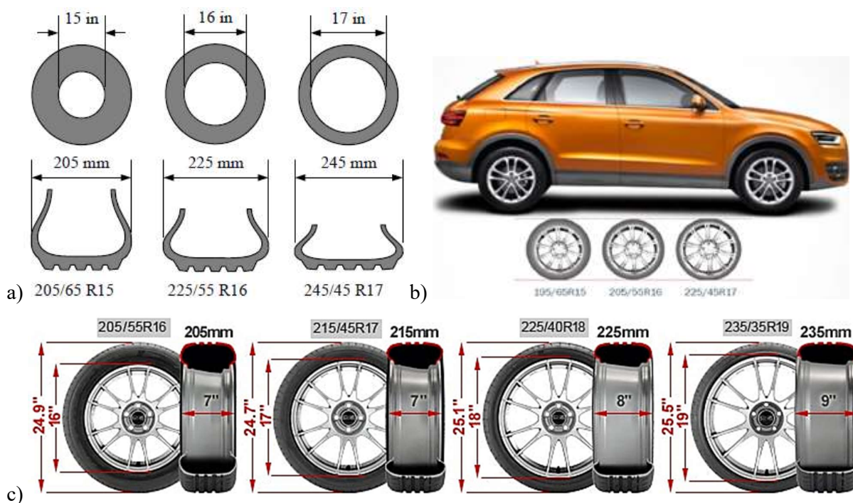
3 pav. Skirtingi padangų matmenys išlaikant tą patį išorinį skersmenį: a) „Plus 1“ koncepcija pritaikyta skirtingų matmenų padangoms (Jazar 2009); b) skirtingų ratų matmenų siūlymas konkrečiam automobiliui ( carwale.com/features/how_tyre_size... ); c) skirtingų ratų matmenų pavyzdžiai ( autoevolution.com/news/bigger-wheels-... )
