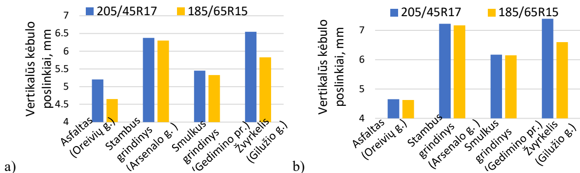
53 pav. Vertikalūs kėbulo poslinkiai pagal skirtingas kelio dangas: a) prie 30 km/h greičio, b) prie 50 km/h greičio
