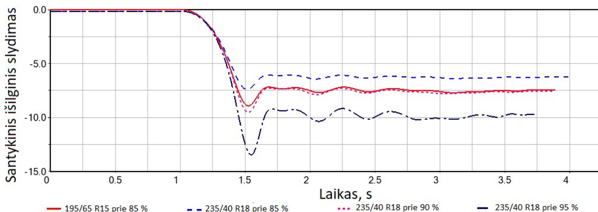
24 pav. Padangos slydimas, tenkantis galiniam kairiajam ratui stabdymo metu
