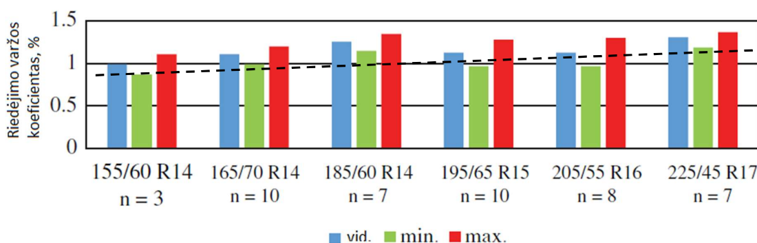
9 pav. Riedėjimo varžos koeficiento priklausomybė procentais nuo vasarinių padangos matmenų (Mauwerk 2015)
