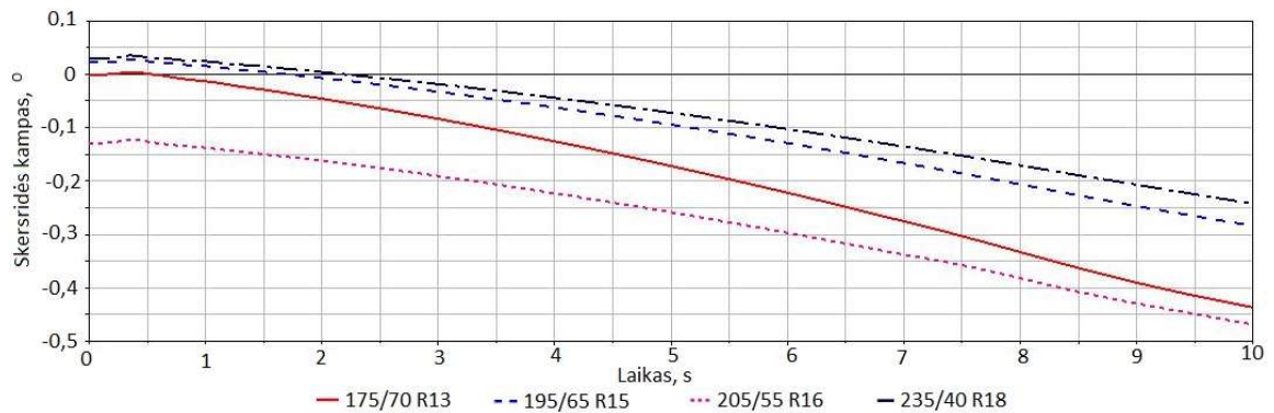
40 pav. Skersridės kampas posūkio metu, kada posūkio spindulys yra pastovus
