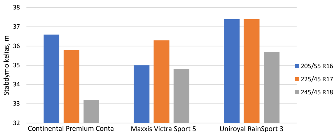
18 pav. Auto Bild ekspertų atliktų testų rezultatai stabdant 100–0 km/h ant sausos dangos
