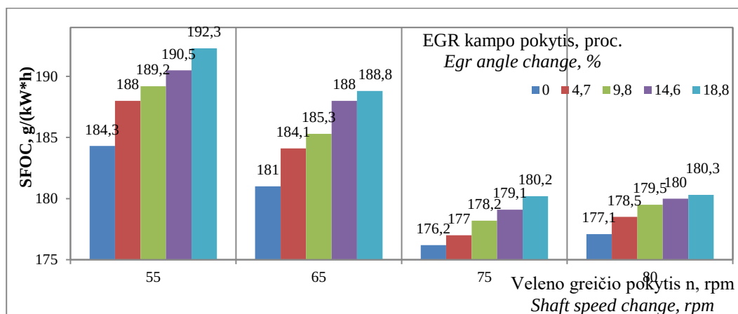
3 pav. Jūrų dyzelinio variklio specifinio kuro sąnaudų pokyčiai Fig.3 Changes in the specific fuel consumption of a marine diesel engine
