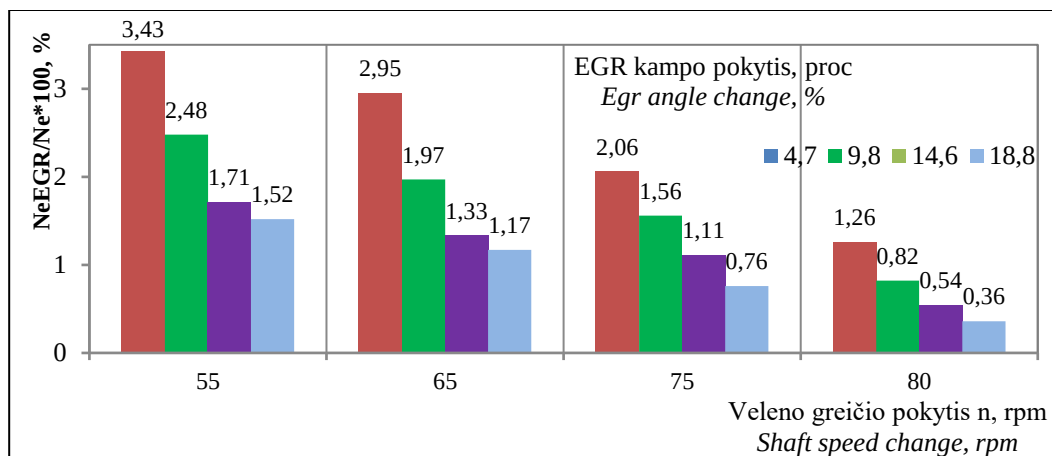
4 pav. Santykinis galios praradimas jūriniame dyzeliniame variklyje Fig.4 Relative power loss in a marine diesel engine
