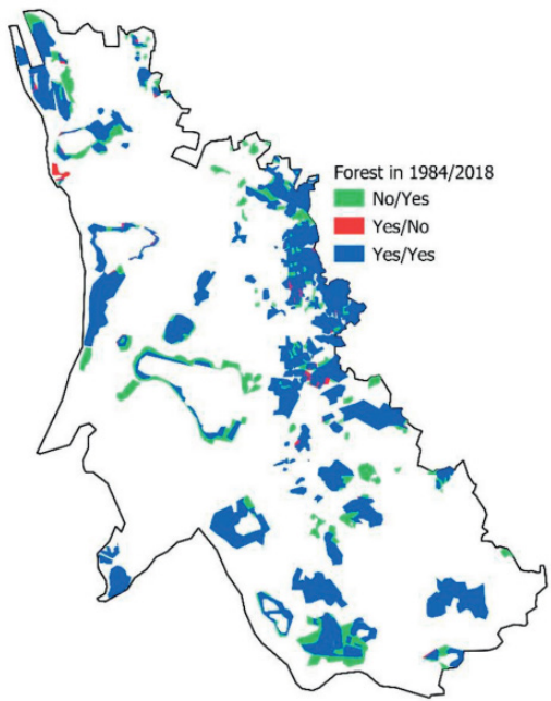
3.3 pav. Miško išplitimo teritorijos nuo 1984 iki 2018 m. pagal Gozdowski ir kt. 2020.
