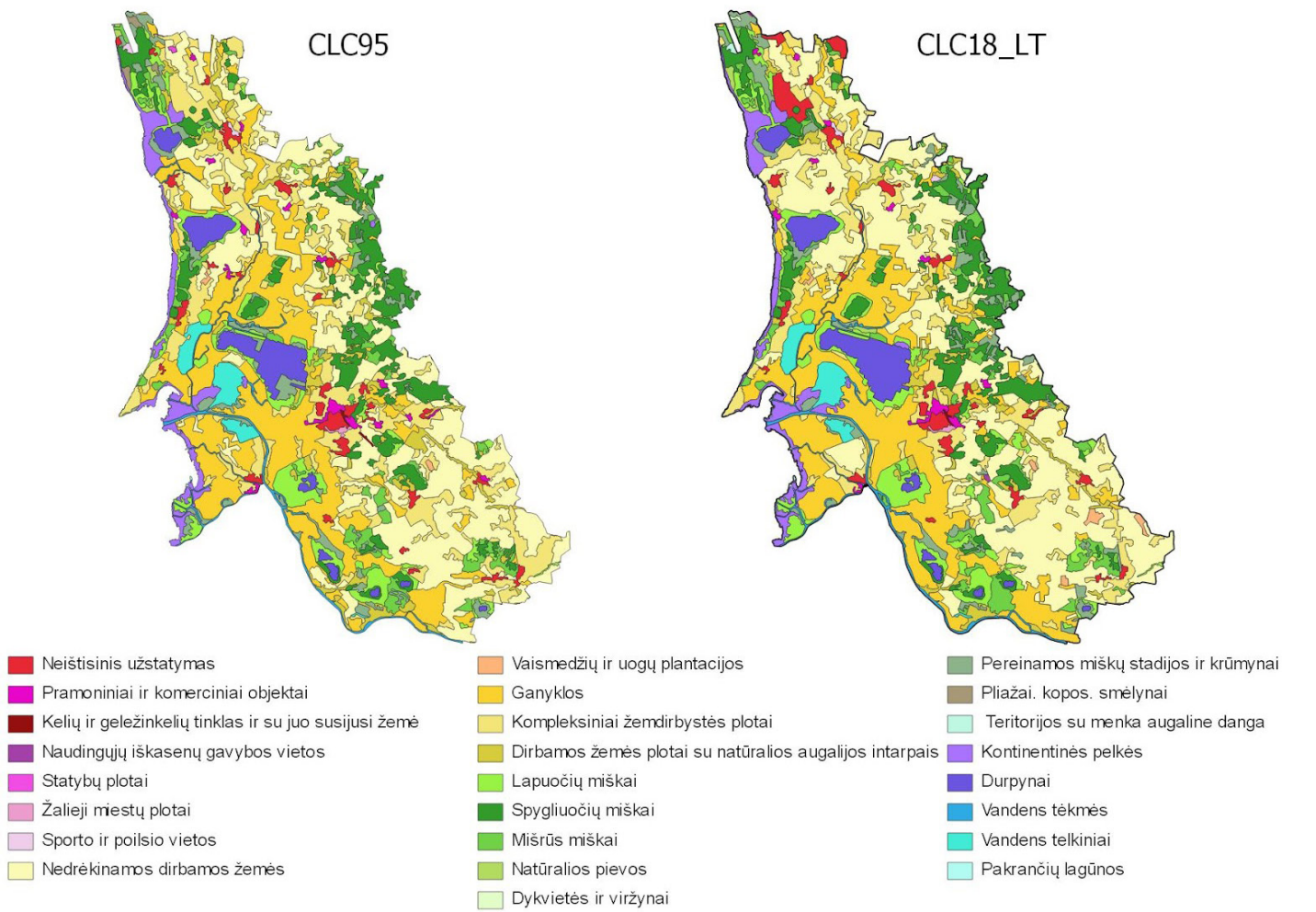
3.4 pav. Žemėnaudos kaita pagal CORINE (CLC - Corine Land Cover) žemės dangos duomenis 1994-1995 (CLC95) ir 2017 metais (CLC18_LT)
