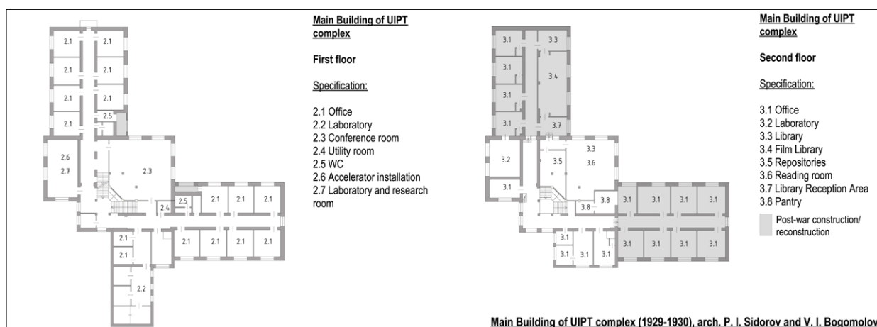
Fig. 5. Main Building, second and third floor plans, by K. Didenko and O. Bondarchuk based on archival NSC KhIPT documents Ryc. 5. Budynek Główny, rzuty pierwszego i drugiego pietra; opr. K. Didenko i O. Bondarczuk na podstawie dokumentów archiwalnych NCN ChIFT
