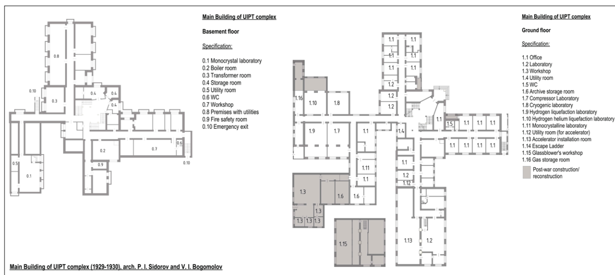
Fig. 4. Main Building, basement and first floor plans; by K. Didenko and O. Bondarchuk based on archival NSC KhIPT documents Ryc. 4. Budynek Główny, rzuty piwnic i parteru; opr. K. Didenko i O. Bondarczuk na podstawie dokumentów archiwalnych NCN ChIFT
