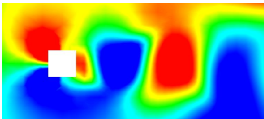
2.17 pav. Periodiniai sūkuriai už kvadratinio skerspjūvio (dažnis 1,1 Hz)
