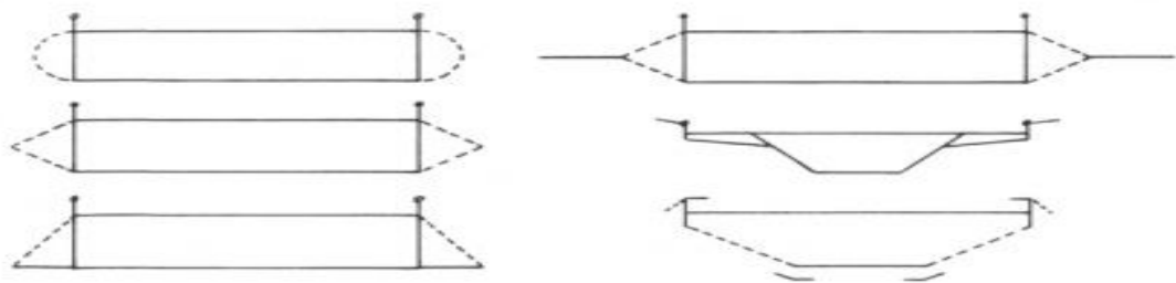
4.8 pav. Standumo sijų aptakai [10].
