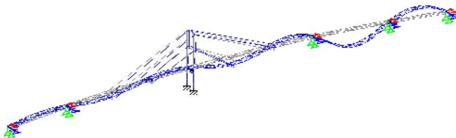
3.5 pav. Vantinio tilto vertikalųjų svyravimų forma (2,781 Hz)
