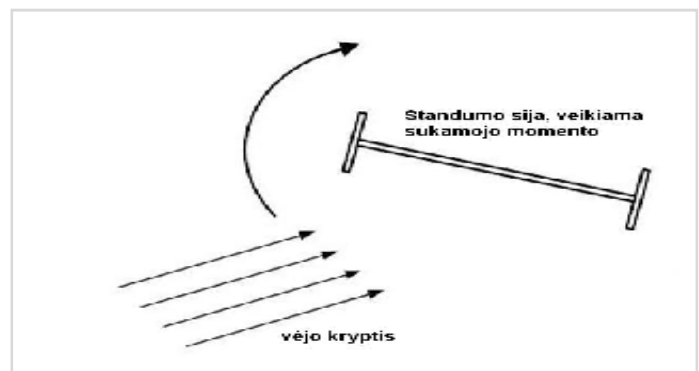
2.23 pav. Siją veikiamą neigiamos krypties sukimo momento [30]
