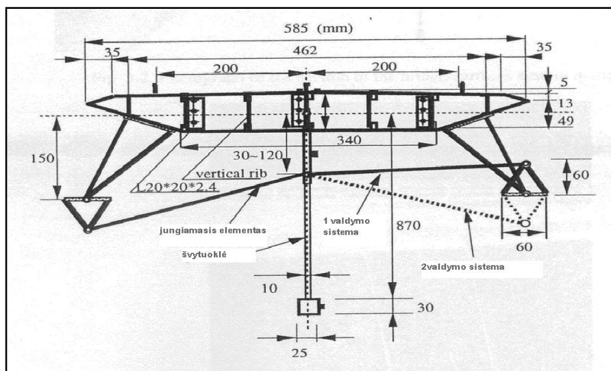
4.28 pav. Veikiančio pasyvaus standumo sijos slopintuvo modelio schema [18]
