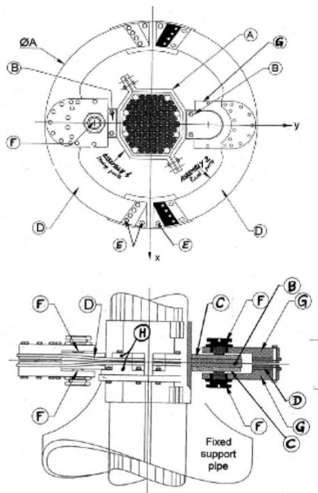
4.26 pav. Trinties slopintuvo schema [12]
