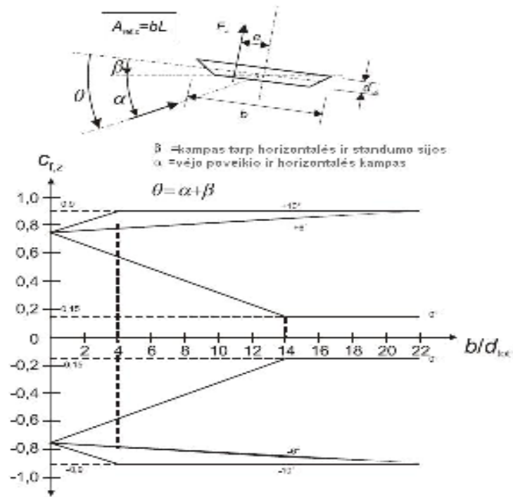
2.7 pav. Jėgos koeficientai
