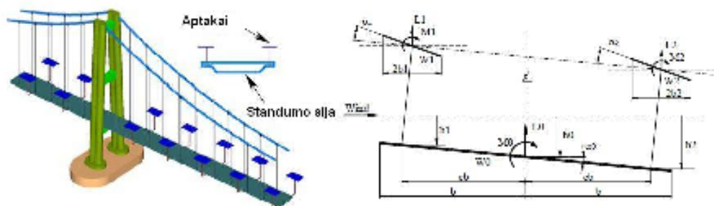
4.42 pav. Standumo sija su kitokiu aptakų tvirtinimu [18]
