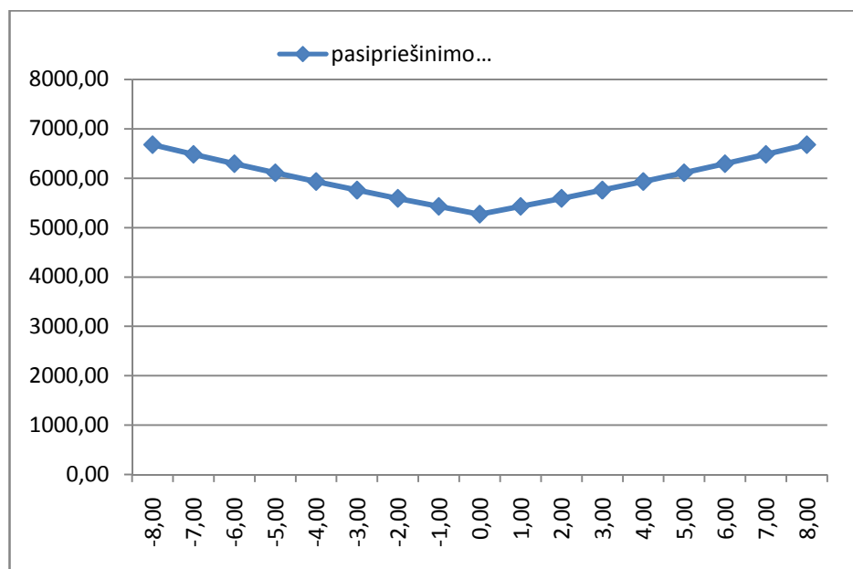
3.3 pav. Pasipriešinimo jėgos grafikas, esant kintamam vėjo atakos kampui (nuo -8° iki +8°)
