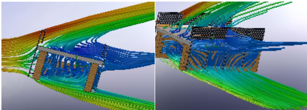
3.7 pav. Vėjo tėkmės izolinijos a) izolinijos apie skerspjūvį, b) izolinijos už skerspjūvio
