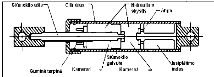
4.18 pav. Realus hidraulinio slopintuvo pjūvis
