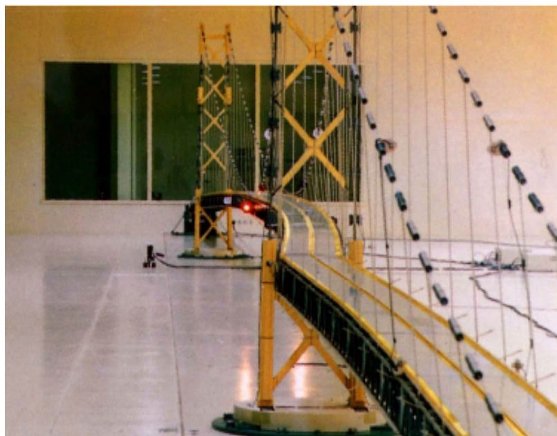
1.16 pav. Akashi Kaikyo tilto modelis aerodinaminiam vamzdyje, pučiant 90 m/s dirbtiniam vėjui [33]
