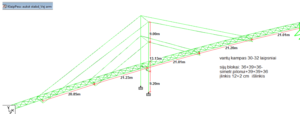
3.1 pav. Vantinio tilto schema
