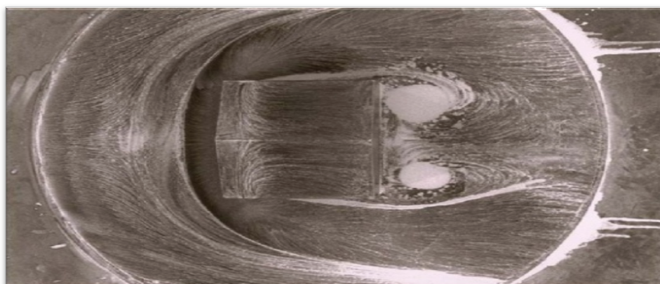
2.15 pav. Klampaus skysčio tėkmė už skerspjuvio
