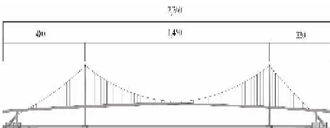
4.36 pav. Modeliuojamo Gwangyang tilto schema
