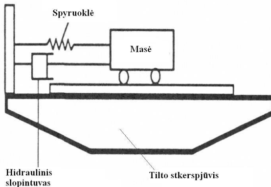
4.9 pav. Masės slopintuvo principinė schema
