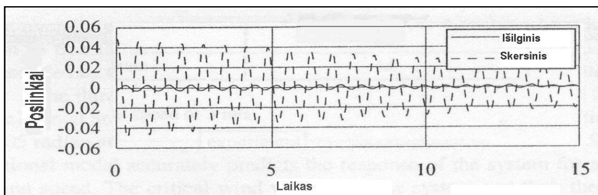
4.29 pav. Išilginis ir skersinis sijos poslinkiai prie 3 m/s vėjo greičio, kai sijos modelio skerspjuvis be aptakų [18]
