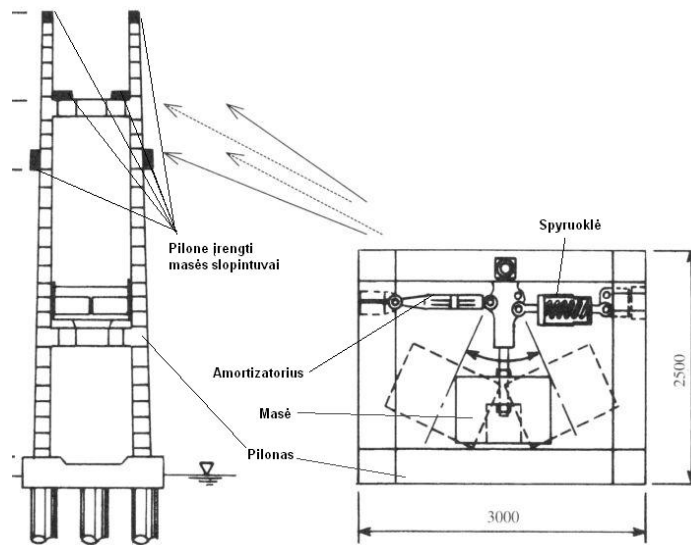
4.11 pav. Slopintuvai pilonuose
