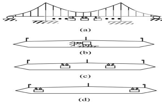
4.10 pav. Trijų virpėjimo krypčių masės slopintuvai: a) taškai, kuriuose įrengiami slopintuvai, b) horizontalios, c) vertikalios, d) sukamos [10]
