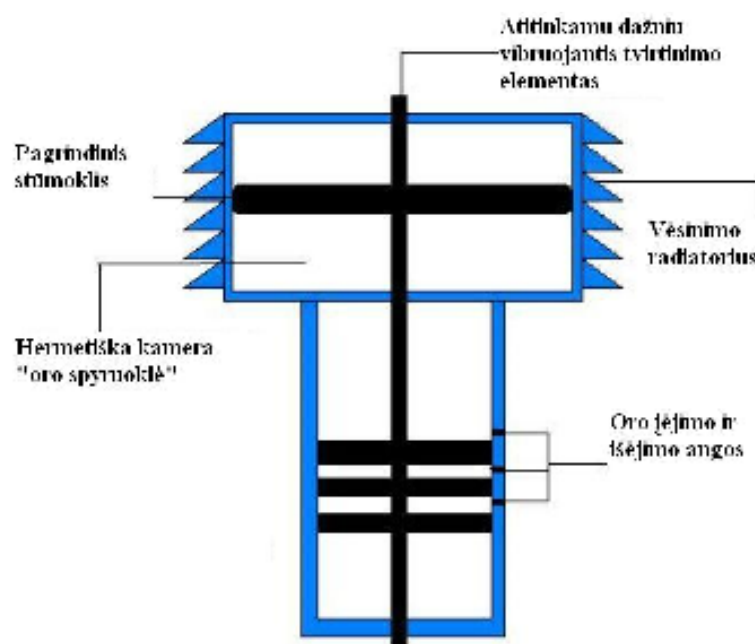
4.1 pav. Tesla virpesių generatorius
