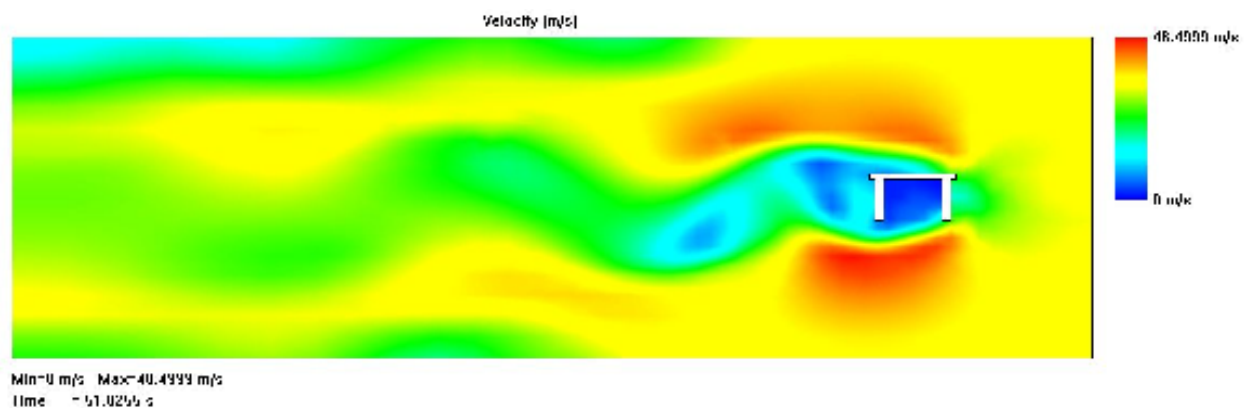
3.10 pav. Periodiniai sūkuriai už tilto skerspjuvio
