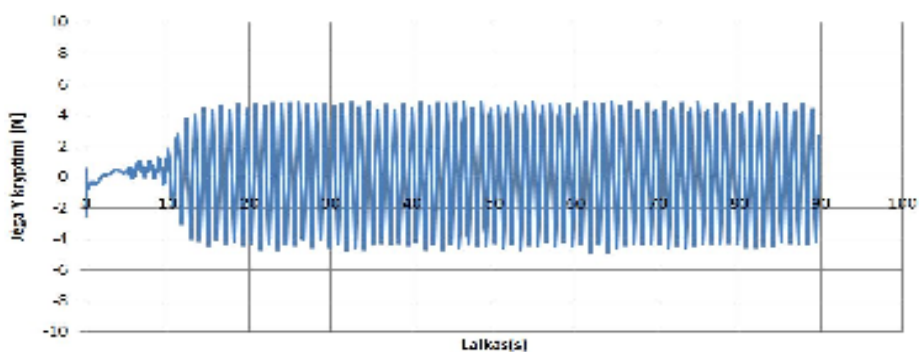
2.18 pav. Jėgos, dėl periodinių sūkurių, kitimo grafikas laike
