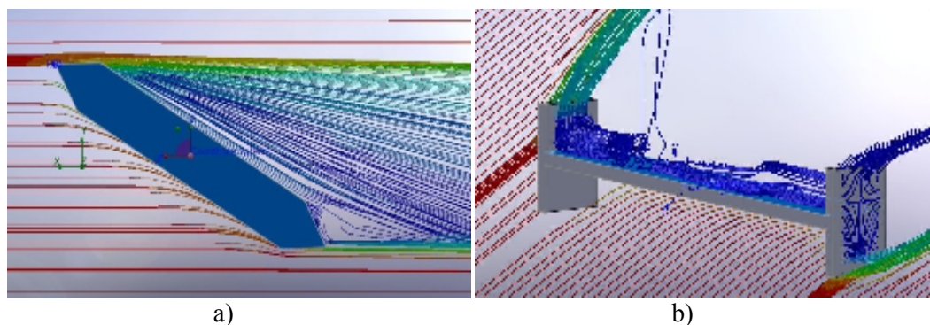
2.27 pav. Skerspjūvių aptakumą vaizduojančios izolinijos a) aptakaus skerspjūvio, b) H tipo skerspjūvio.
