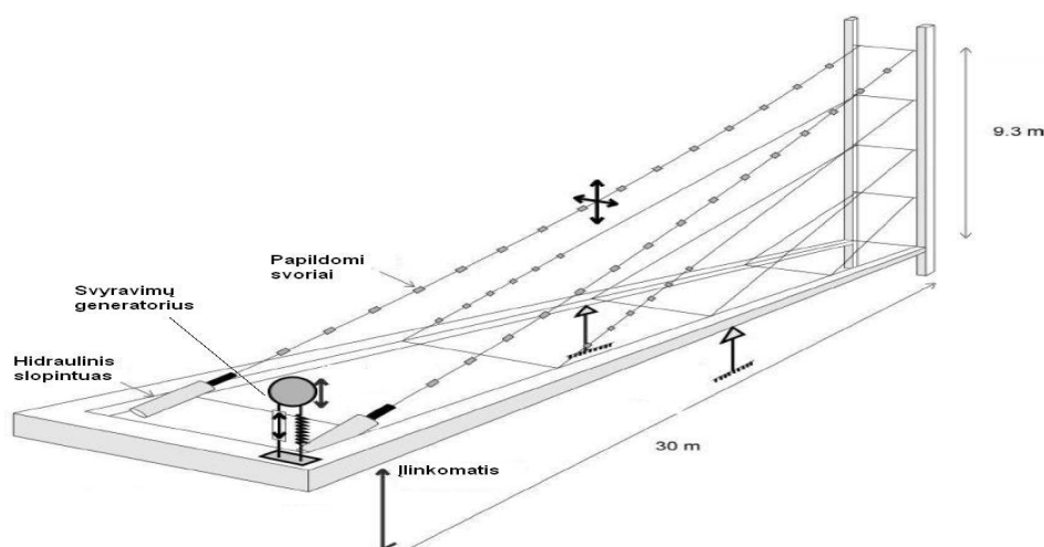
4.33 pav. Dresdeno universiteto laboratorijoje pagamintas vantinio tilto modelis
