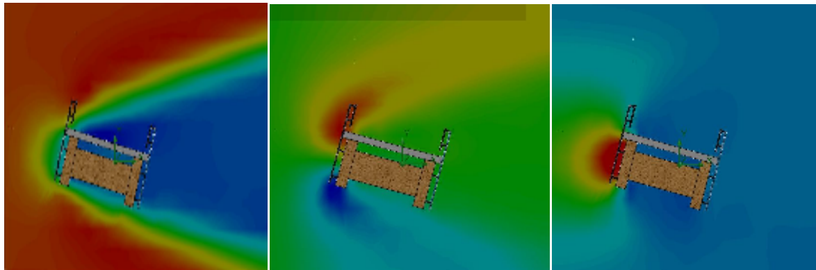
a) b) c) 3.8 pav. Vėjo srautas apie standumo siją -30^\circ kampu a) srauto greitis horizontalia (x kryptimi), b) srauto greitis vertikalia (y kryptimi) c) vėjo slėgis
