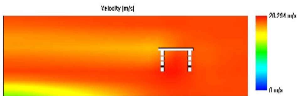
4.46 pav. Standumo sija su šonuose įrengtom angom.
