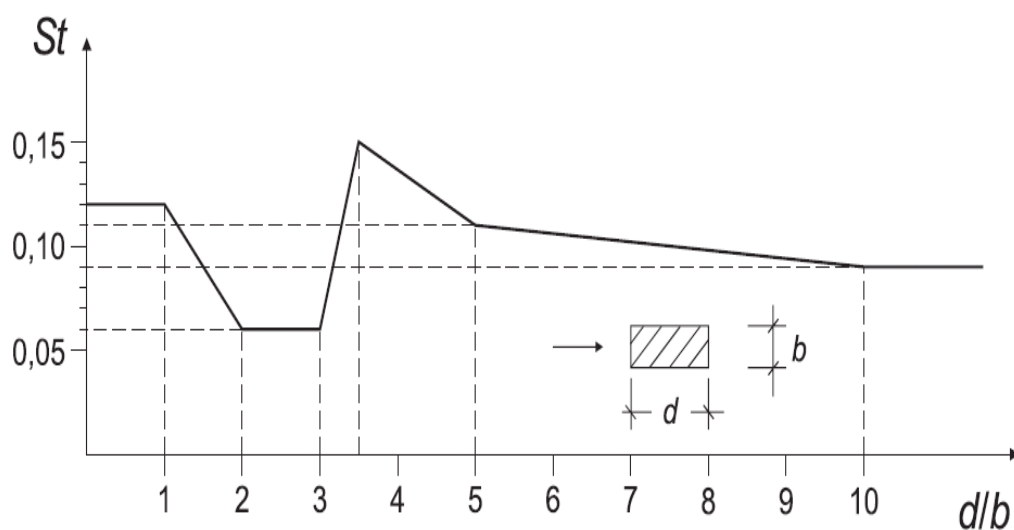
2.16 pav. Stačiakampių skerspjūvių aštriais kampais Strouhalo ( St ) skaičius
