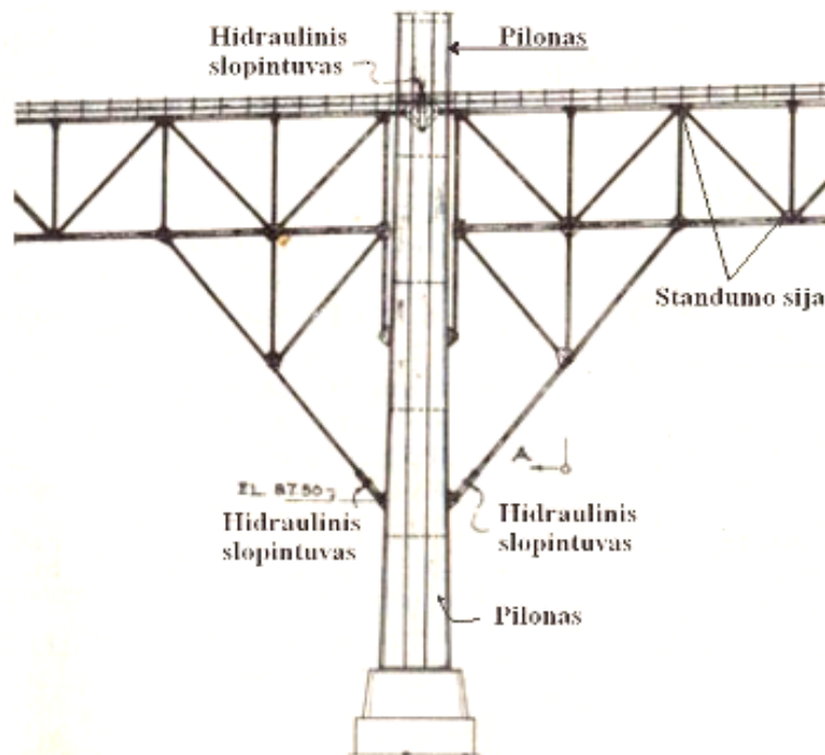
4.24 pav. Naujojo Tacoma Narrows tilto st. sijos jungimas su pilonu per slopintuvus [34]
