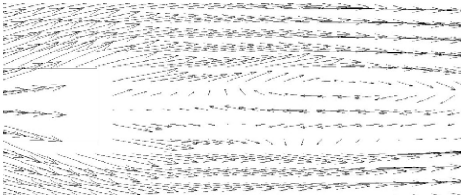
2.14 pav. Oro tėkmės vektorinė diagrama
