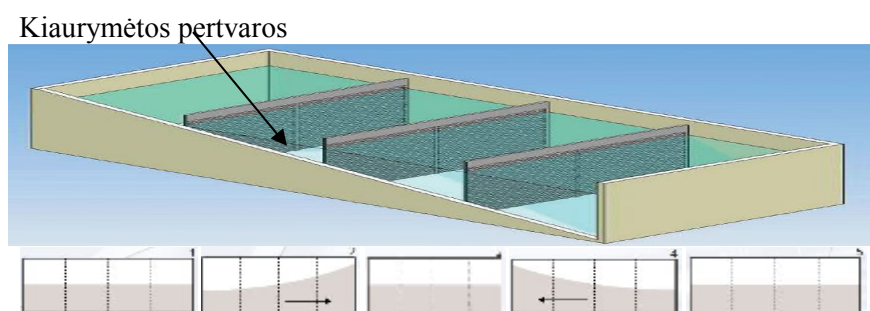
4.12 pav. Pasyvaus teliūskuojančio skysčio slopintuvo principinė schema 1–2–3–4–5 skysčio judėjimas esant horizontaliems siūbavimams
