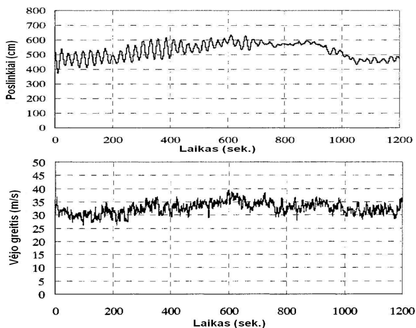
1.8 pav. Akashi Kaykio tilto poslinkiai ir vėjo greičiai 1998 metais siautuso taifūno metu [33]
