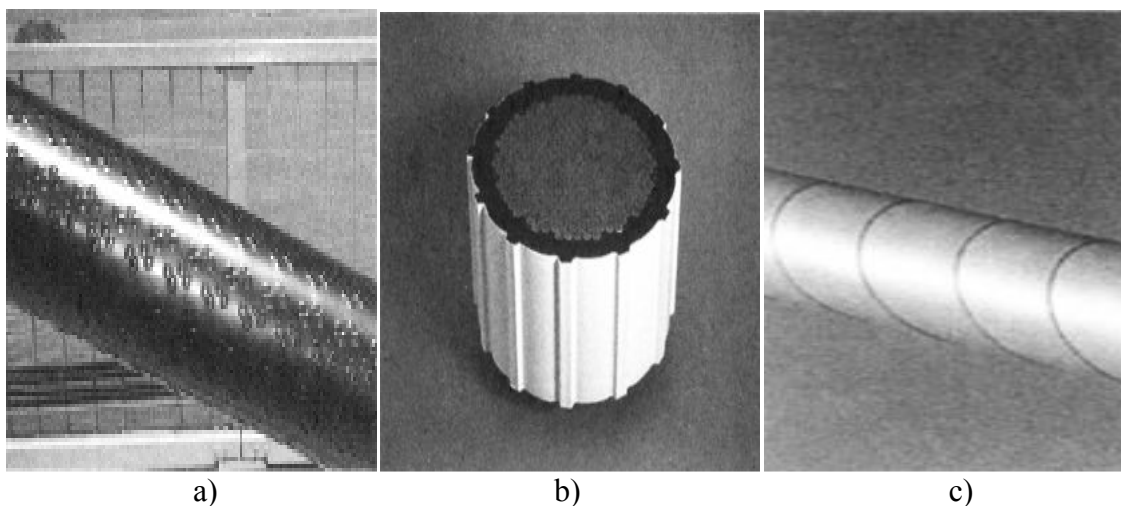
4.7 pav. a) Lyno paviršiuje padarytos duobutės Tataru tiltas Japonijoje; b) Įrengtos iškilusios juostelės lygiagrečios lynui Higashi–Kobe tilte Japonijoje; c) spiralės formos iškilimai Vasco de Gama tilte Portugalijoje [10]
