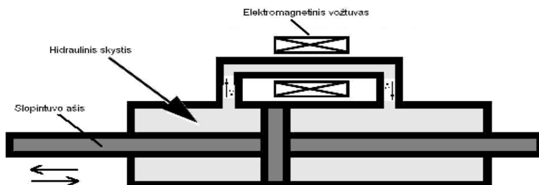
4.32 pav. Principinė aktyvaus hidraulinio slopintuvo schema
