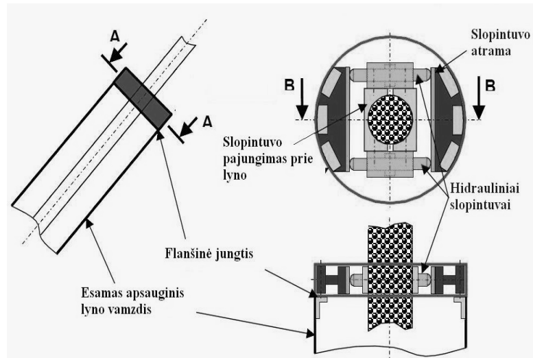
4.22 pav. Kitokio tipo vantų hidrauliniai slopintuvai [2]
