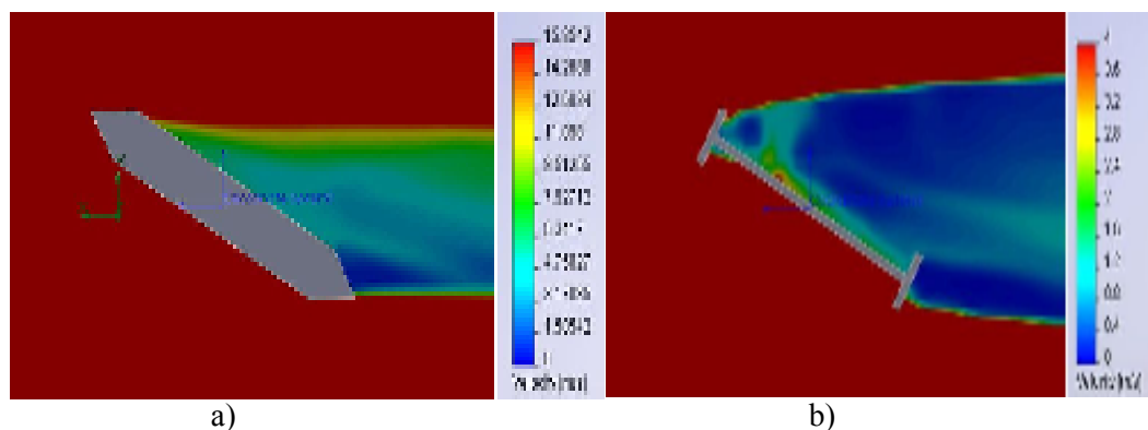
2.26 pav. Nufiltruotos vėjo greičių spalvinės diagramos už skerspjūvių a) aptakaus skerspjūvio, b) H tipo skerspjūvio
