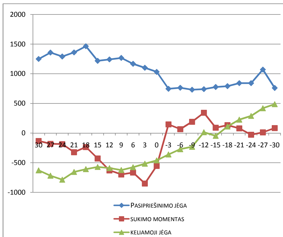
3.9 pav. Pasipriešinimo, keliamosios jėgų ir sukimo momento grafikai, vėjui veikiant 1 tiesinį metrą standumo sijos nuo -30^\circ iki +30^\circ vėjo atakos kampui
