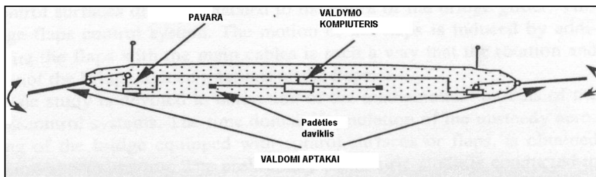
4.41 pav. Aktyvaus standumo sijos slopintuvo aptakais principinė mechaninė schema [18]
