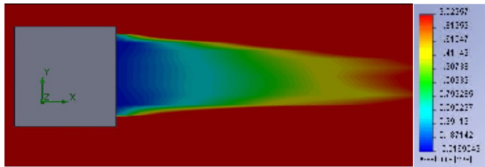
2.10 pav. Nufiltruotas minimalaus greičio, srauto judėjimas už bukojo skerspjūvio x kryptimi
