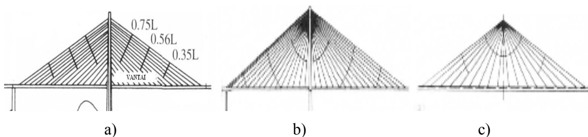
4.4 pav. a) Faro tiltas Danijoje, b) Helgeland tiltas Norvegijoje, c) Yobuko tiltas Japonijoje [10]
