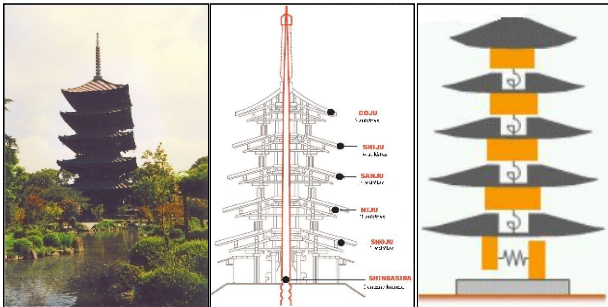
4.2 pav. Budistų šventyklų Pagoda vaizdai: a) bendras budistų šventyklos Pagoda vaizdas; b) Šventyklos principinė schema; c) Šventyklos skaičiuojamoji schema [16]
