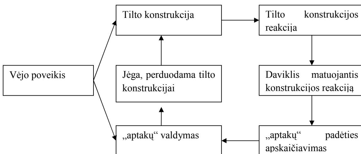
4.40 pav. Aktyvaus, aerodinaminio poveikio, slopintuvo principinė valdymo schema
