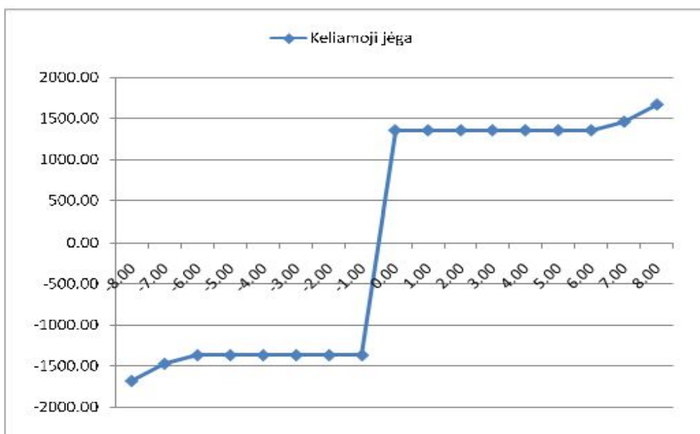
3.4 pav. Keliamosios jėgos grafikas esant kintamam vėjo atakos kampui (nuo -8^\circ iki +8^\circ )
