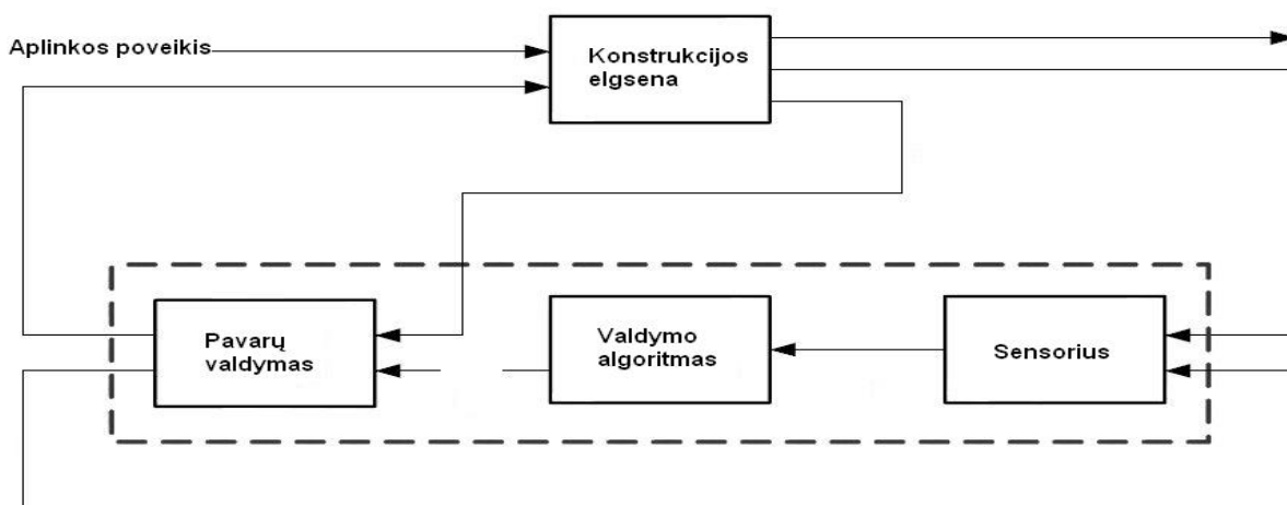
4.31 pav. Aktyvios slopinimo sistemos veikimo schema
