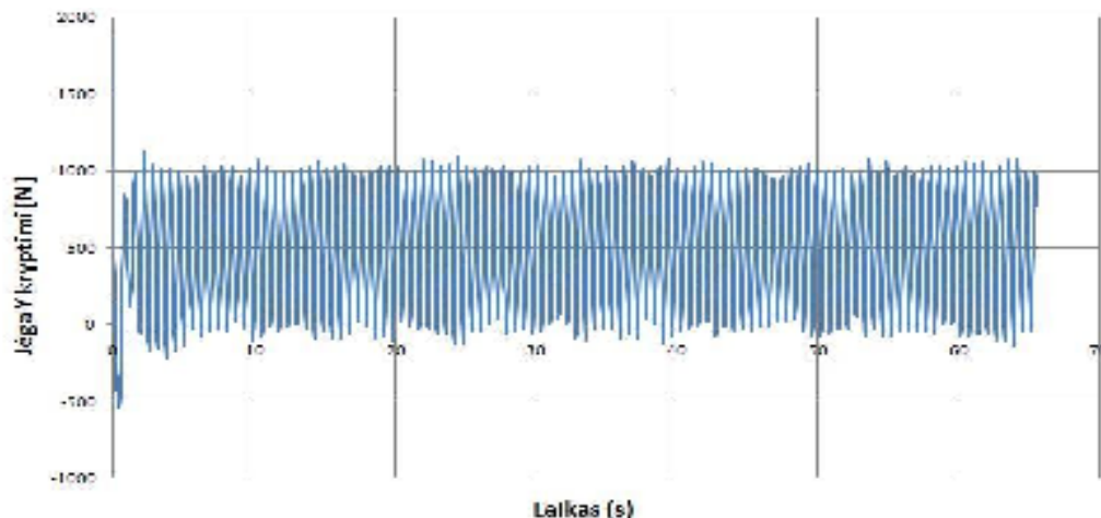
3.10 pav. Periodiniai sūkuriai už tilto skerspjuvio
