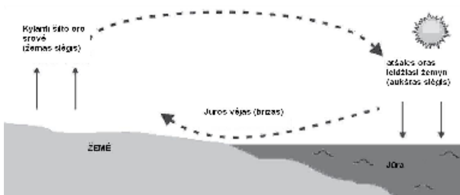
1.12 pav. Ryšys tarp aušto ir žemo atmosferos slėgio dieną
