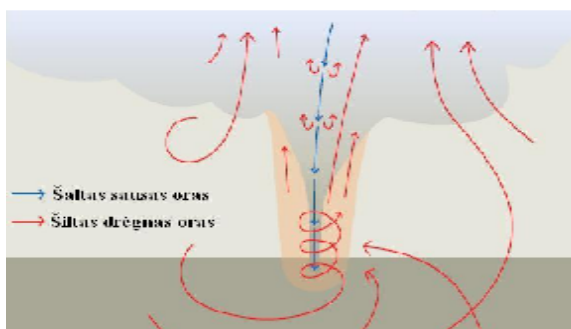
1.14 pav. Tornado susidarymo schema
