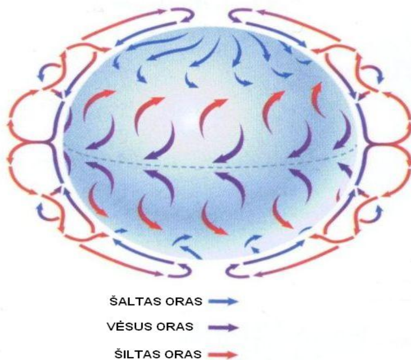
1.11 pav. Oro srauto judėjimo kryptys apie žemės paviršių dėl Koriolio efekto.
