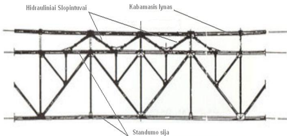
4.23 pav. Naujojo Tacoma Narows tilto lyno jungimas su standumo sija per slopintuvus [34]
