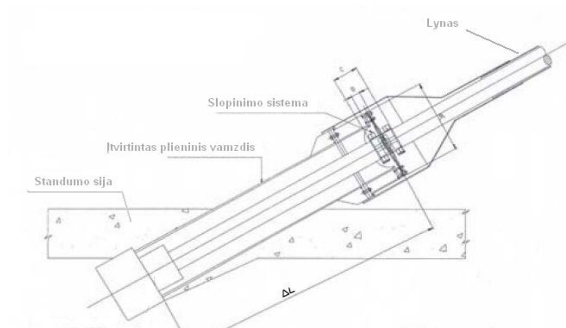
4.27 pav. Lyno ir trinties slopintuvo tvirtinimo mazgas
