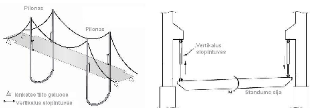
4.35 pav. Hidrauliniai slopintuvai, skirti plazdėjimo sukeltiems sukamiesiems svyravimams standumo sijoje slopinti
