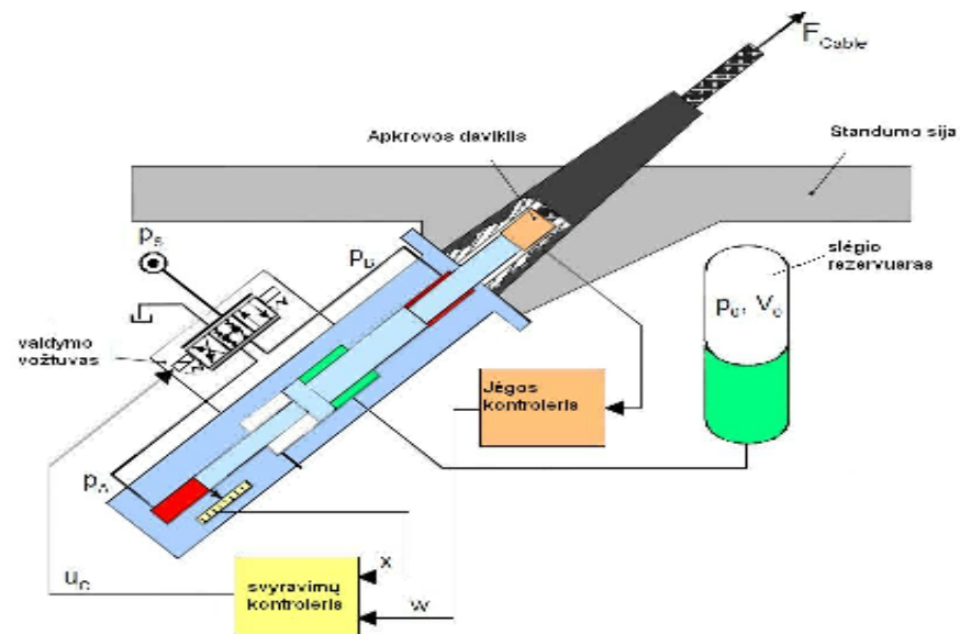
4.34 pav. Dresdene bandyto slopintuvo schema
