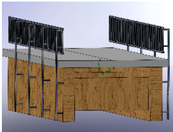
3.6 pav. Modeliuotas 6 m ilgio vantinio tilto standumo sijos skerspjūvis
