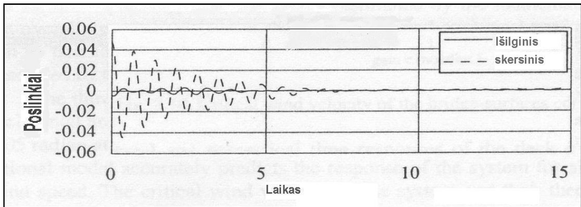
4.30 pav. Išilginis ir skersinis sijos poslinkiai prie 3 m/s vėjo greičio, kai sijos modelio skerspjuvis su aptakais [18]
