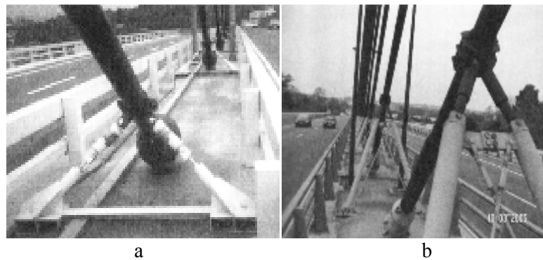
4.19 pav. Hidrauliniai vantų slopintuvai: a) Aratsu tiltas Japonijoje b) Iroise tiltas Prancūzijoje hidrauliniai [10]
