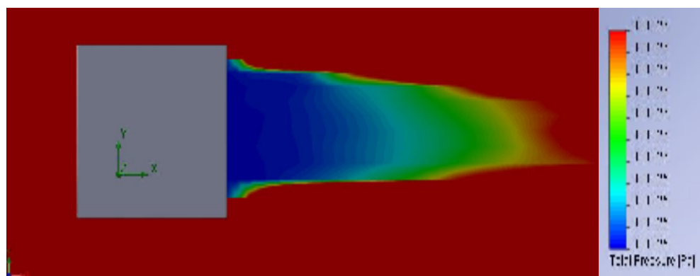
2.12 pav. Sumodeliuoto bukojo skerspjūvio sraute slėgio pasiskirstymo diagrama
