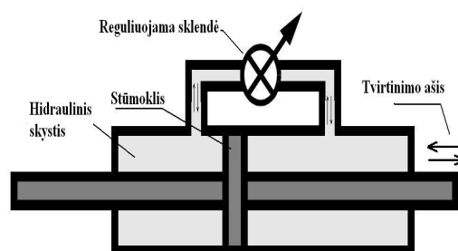
4.17 pav. Principinė reguliuojamo hidraulinio slopintuvo schema
