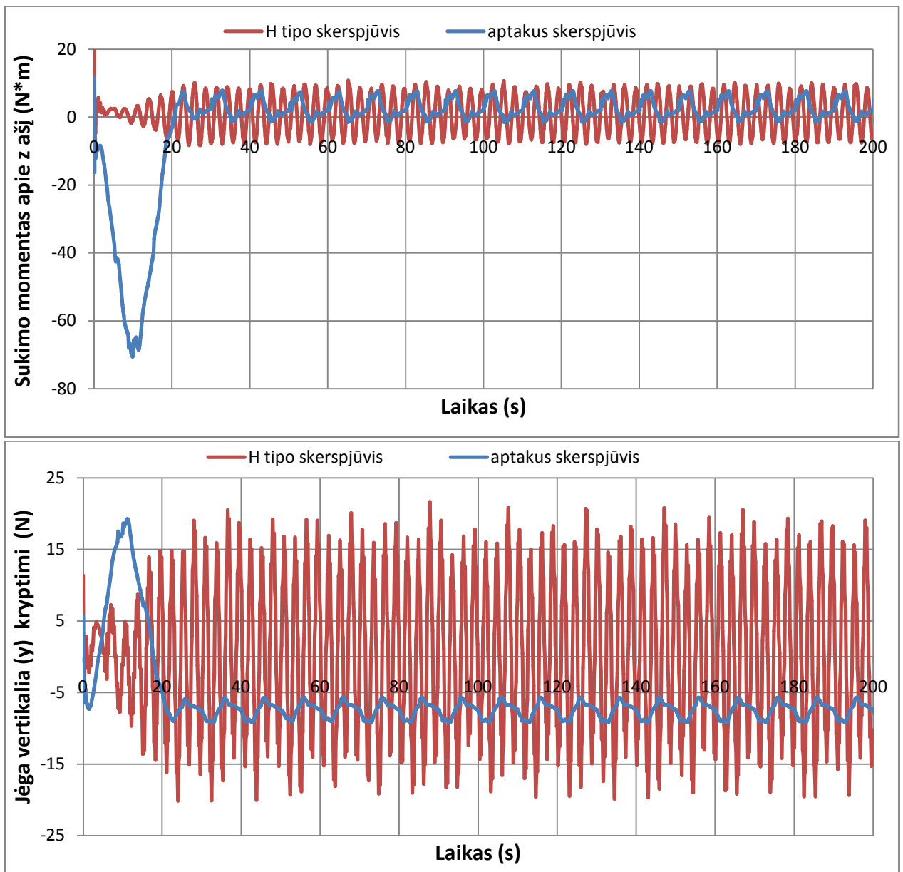
2.20 pav. Jėgų kitimo grafikai, H tipo ir aptakiame skerspjūviuose, veikiant periodiniams sukuriams
