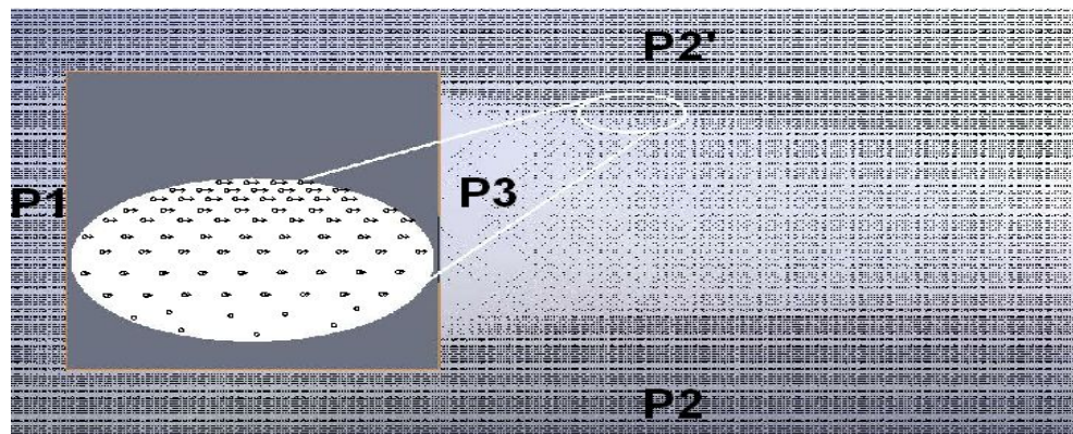
2.11 pav. Grafinis slėgio pasiskirstymo vaizdavimas apie bukąjį skerspjūvį
