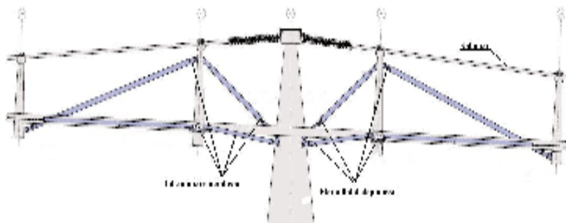
4.21 pav. Hidrauliniai slopintuvai įrengti išilgai Millenium tilto skerspjūvio
