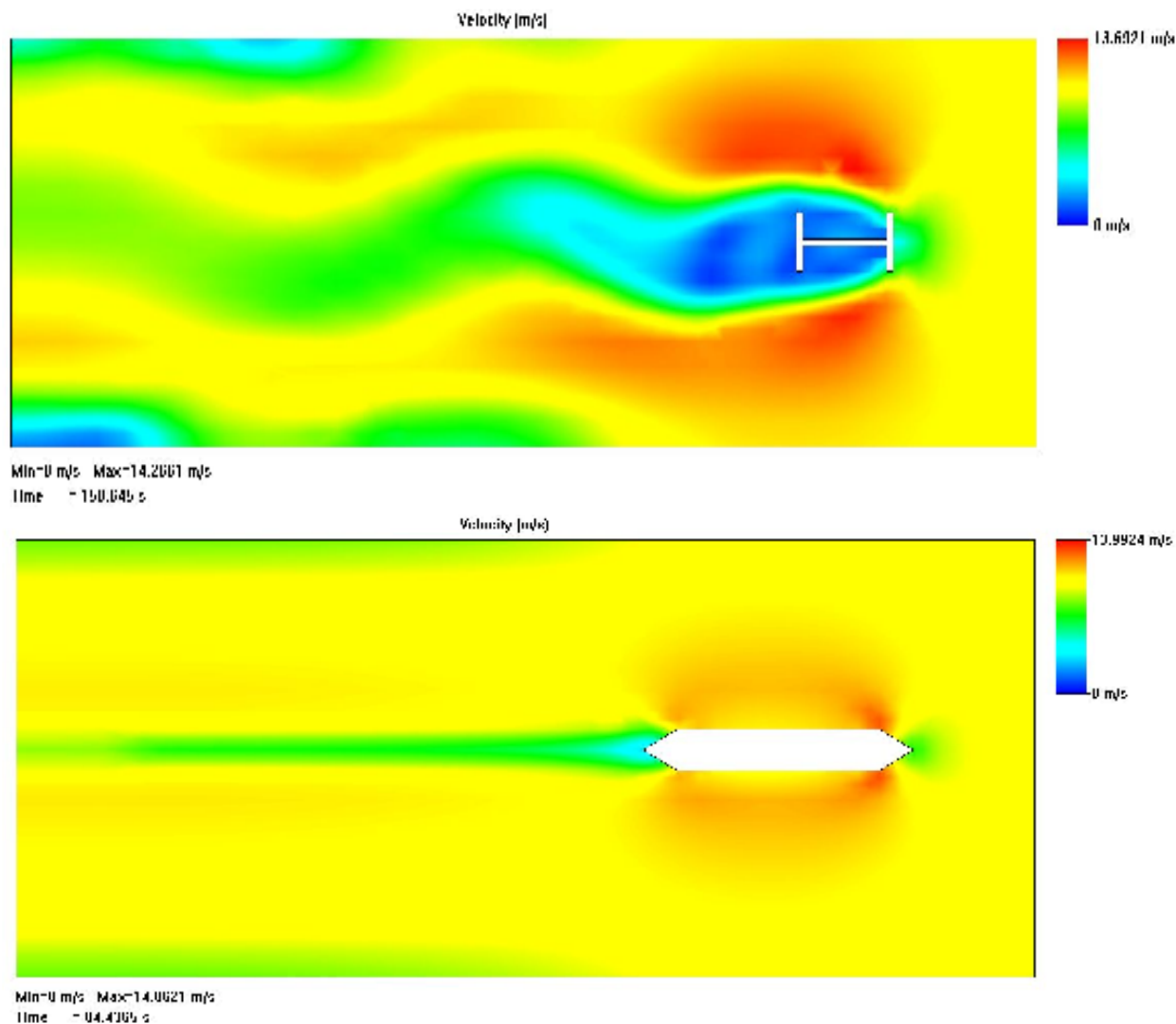
2.21 pav. Tėkmės greičių pasiskirstymo spalvinės diagramos apie nagrinėjamus skerspjūvius
