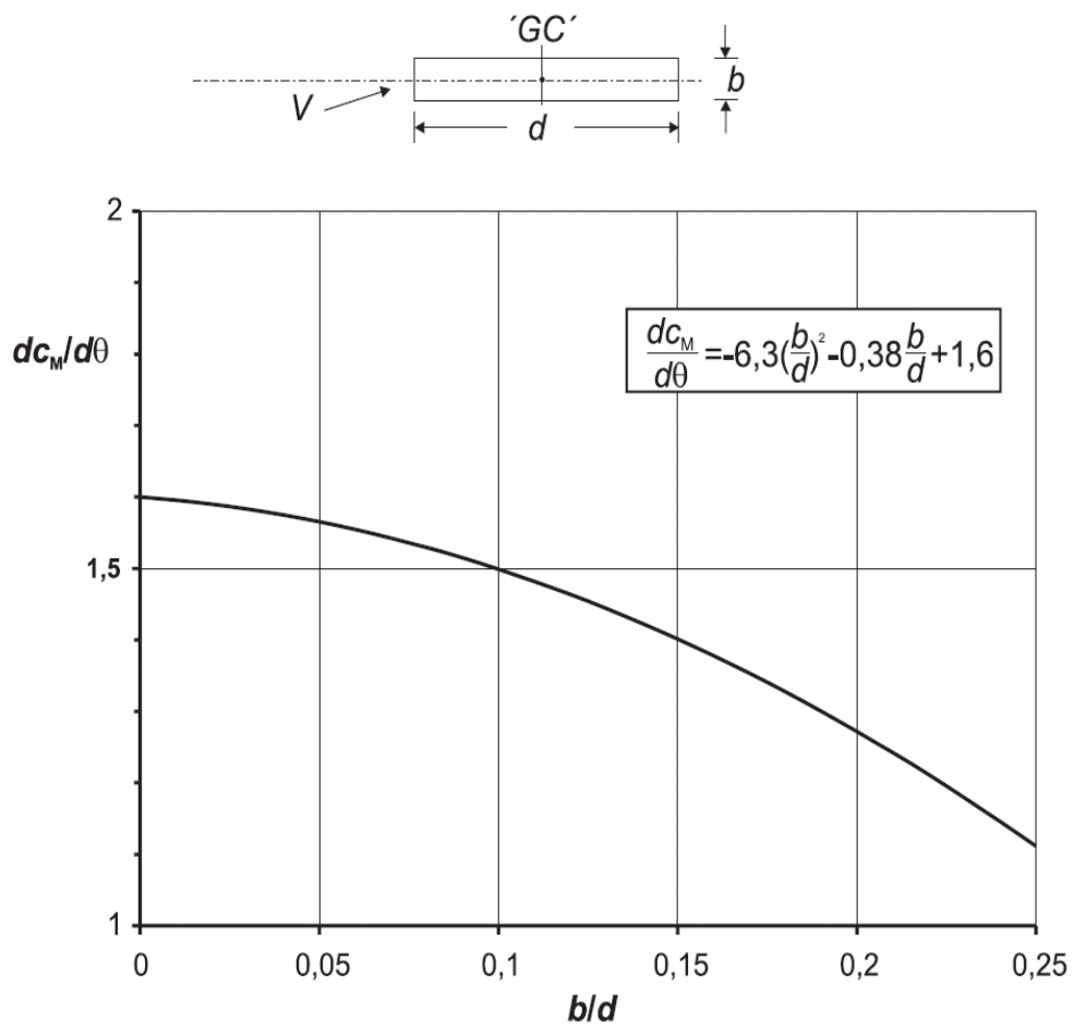
2.29 pav. Aerodinaminio momento (geometrinio svorio centro 'GC' atžvilgiu) koeficiento c_M kitimo spartos priklausomybė nuo \theta , išreikšto b/d [21].
