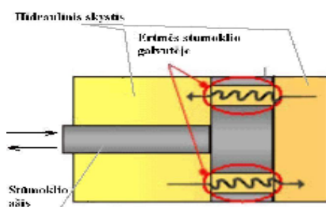
4.16 pav. Principinė pasyvaus hidraulinio slopintuvo veikimo schema
