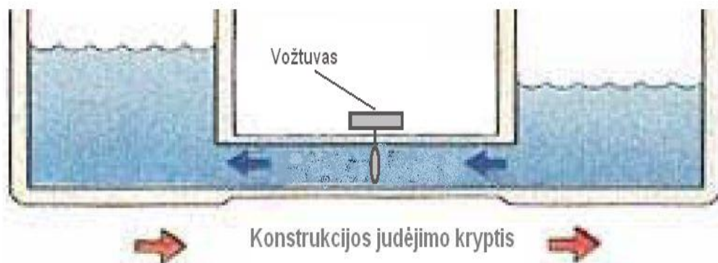
4.39 pav. Aktyvaus, valdomo vožtuvu skysčio slopintuvo schema
