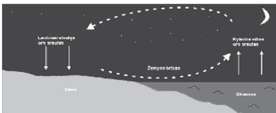
1.13 pav. Ryšys tarp aušto ir žemo atmosferos slėgio naktį
