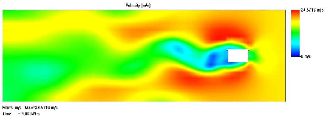
4.44 pav. Vėjo greičių apie skerspjūvį pasiskirstymo diagrama, kai modeliui priskirtas vėjo greitis yra 18m/s
