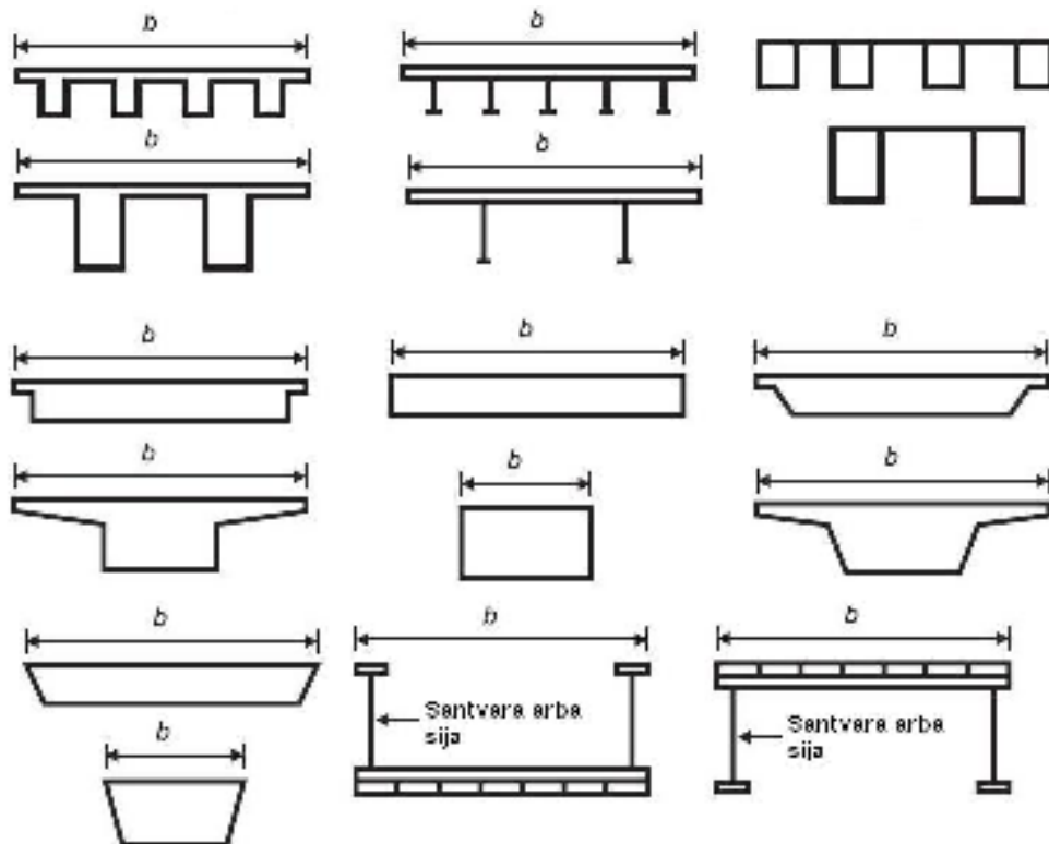
2.1 pav. Įprastinių standumo sijų skerspjūviai
