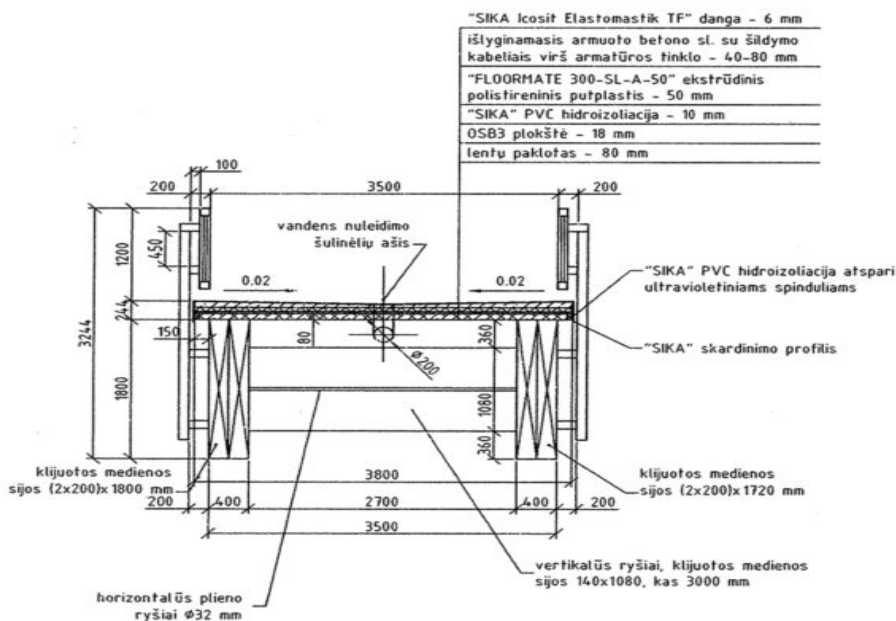
3.2 pav. Vantinio tilto standumo sijos skerspjūvis
