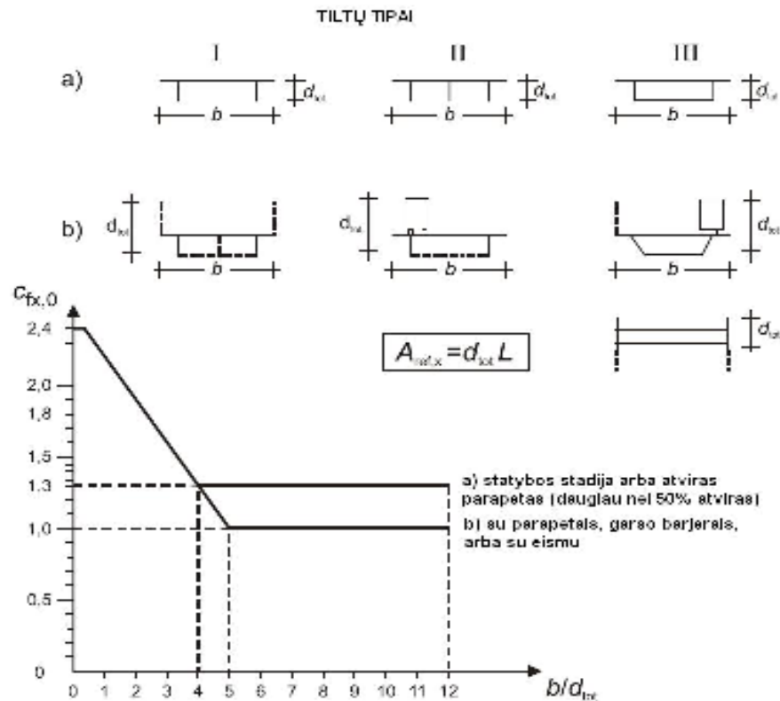
2.5 pav. Tiltų jėgos koeficientai
