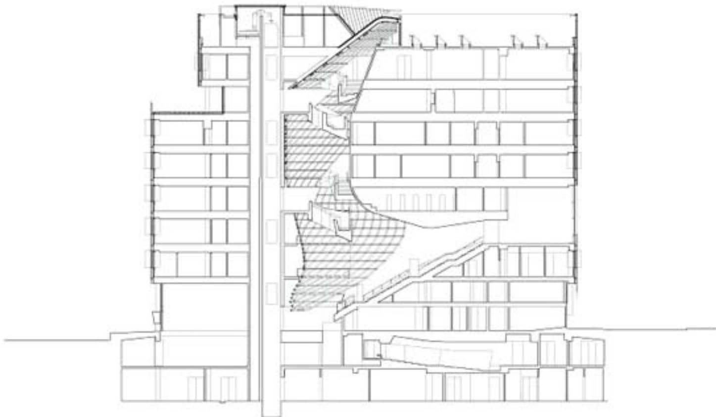
34 pav. Išilginis pastato pjūvis
