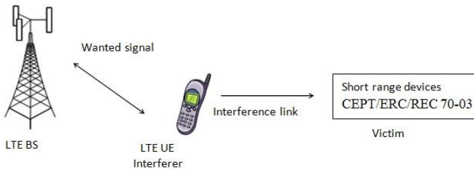
Fig. 2.4. Simulation plan
