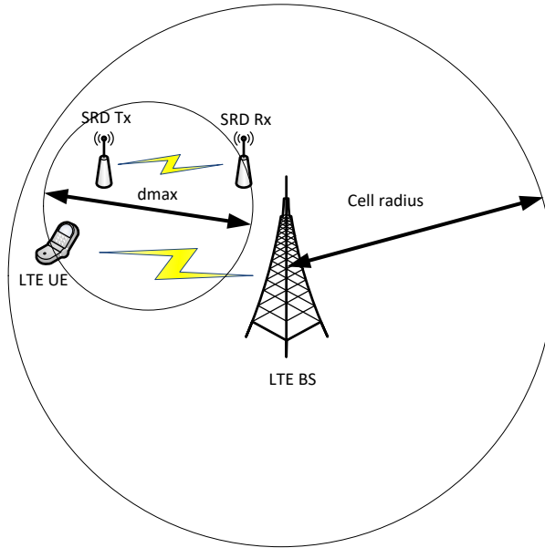
Fig. 2.5. SEAMCAT simulation
