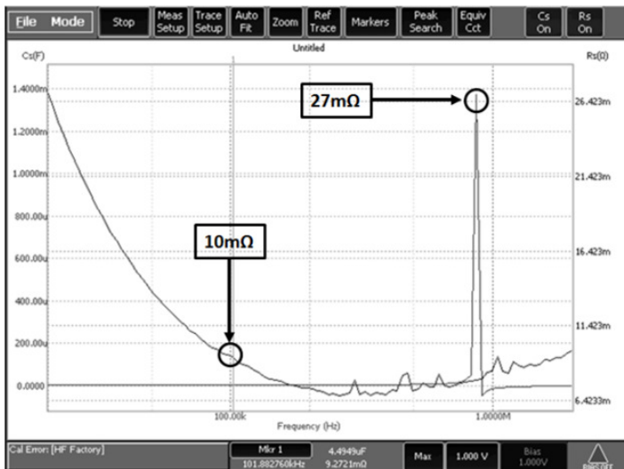
S.4.2 pav. X7R (CKG57NX7R2A106M500JH) kondensatoriaus nuosekliosios ekvivalentinės varžos (NEV) priklausomybė nuo dažnio, kai V_{DC} = 0
