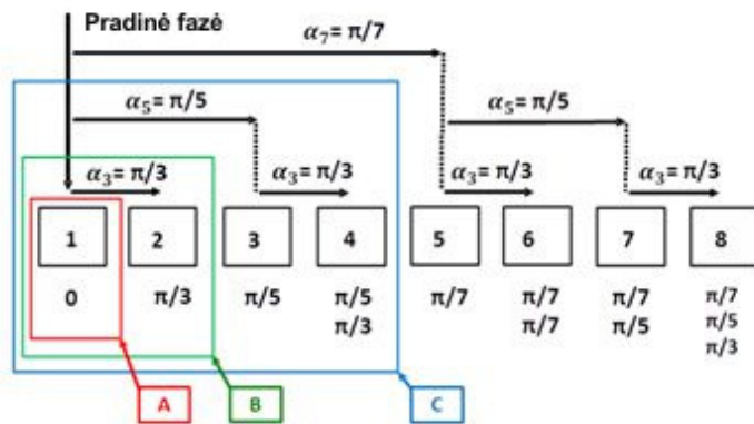
S.5.2 pav. Fazių postūmio algoritmas 3-čios, 5-tos ir 7-tos harmonikos panaikinimui
