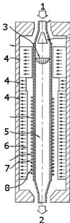
S 2.1 pav. BMR antenos su Faradėjaus ekranu konstrukcijos schematinis brėžinys. 1–2 skysčių įėjimas ir išėjimas, 3 – skysčių srautas, 4 – pastovieji magnetai, 5 – siųstuvo antena (solenoidas), 6 – matavimo kamera, 7 – Faradėjaus ekranas, 8 – siųstuvo-įmtuvo antena
