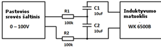
S.4.1 pav. X7R kondensatorių impedanso tyrimo aparatinės įrangos blokinė schema
