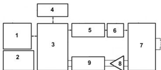
S.5.3 pav. BMR siųstuvo bandymo aparatūros blokinė schema ir signalų perdavimo keliai.
