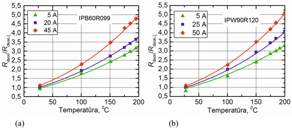
S.3.2 pav. Dviejų skirtingų MOSFET tranzistorių normuotos santakos-ištakos varžos ( R_{\text{dson}}/R_{\text{dson}, I_t} ) priklausomybės nuo temperatūros, esant skirtingoms I_d vėrtėms.
