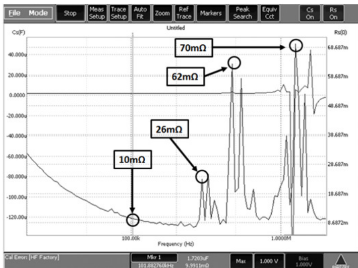
S.4.3 pav. X7R (CKG57NX7R2A106M500JH) kondensatoriaus nuosekliosios ekvivalentinės varžos (NEV) priklausomybė nuo dažnio, kai V_{DC}=50 V
