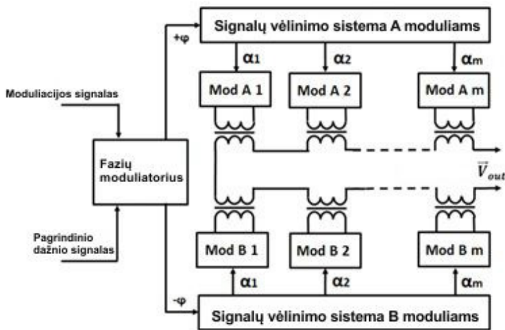
S.5.1 pav. Daugelio modulių BMR siųstovo blokinė schema
