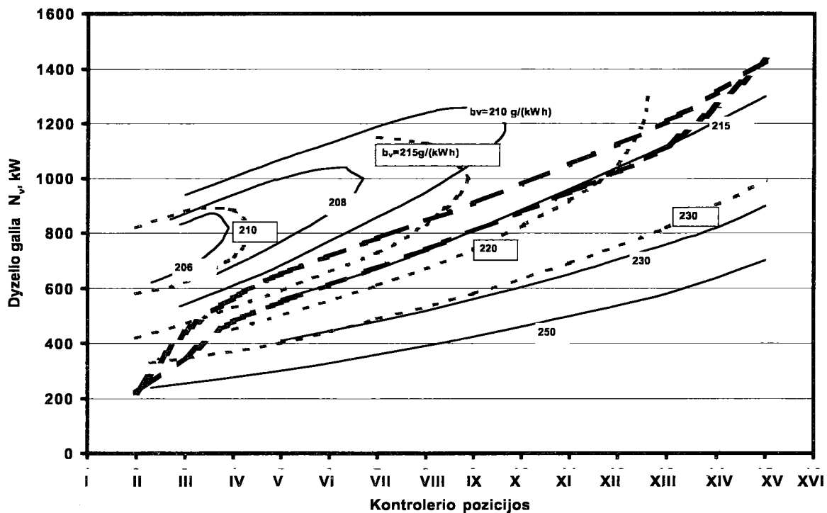
2 pav. 14Д40У2 šilumvežio dyzelio kuro ekonomiškumo sezoniniam darbui padidinimo rezervas, taikant modernizuotas konstrukcijos ASKS (— standartinis ASKS, „žiema“; ---- modernizuotas ASKS, „vasara“)
