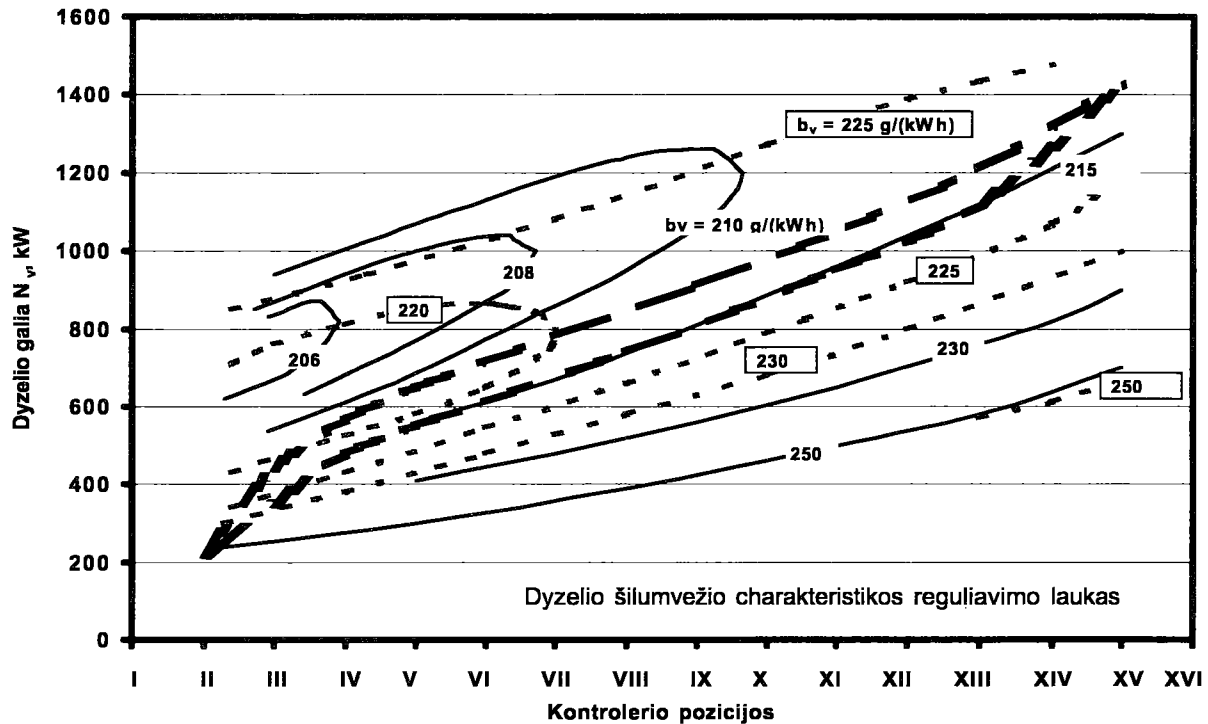
1 pav. Sezono įtaka 14Д40У2 šilumvežio dyzelio specifiniam kuro ekonomiškumui (— „žiema“, T_o = 253\text{ K} ; ---- „vasara“, T_o = 298\text{ K} )
