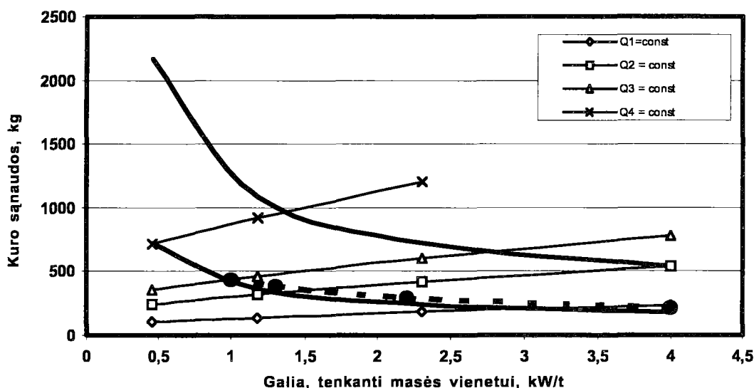
5 pav. Šilumvežio dyzelio 14Д40У2 kuro sąnaudų mažinimas optimizuojant lokomotyvo judėjimo režimą
