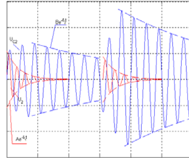
2 pav. Galimos įtampų U_2 ir U_{C2} kitimo kreivės
