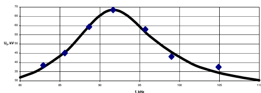
3 pav. Bandymo modelio eksperimento rezonansinė kreivė (pavaizduoti eksperimento taškai ir aproksimuota eksperimento kreivė)
