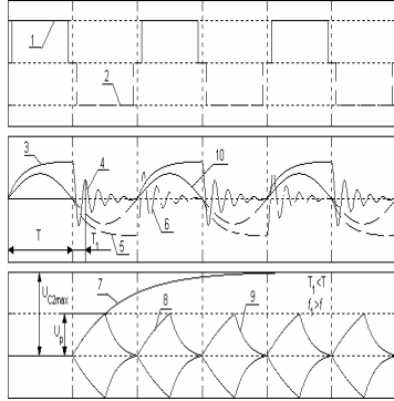
1 pav. Proceso eksperimentinėje schemoje grafikai
