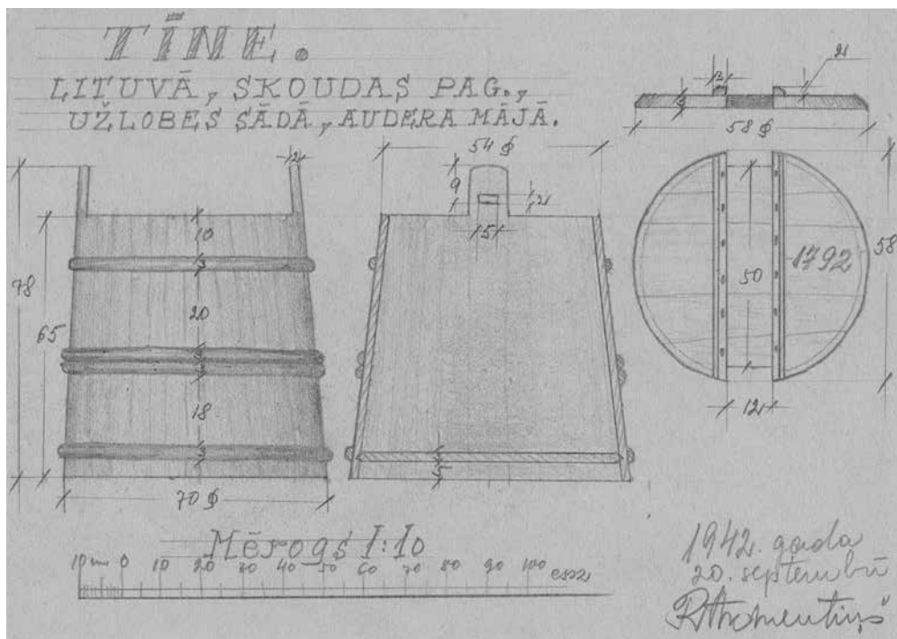
Kraitkubilis, vēlāku laikiem lietots miltams laikītis (tekintu egļu lentas, pušu šakņu lankai), meistars nenustatīts, ant dangčio data – 1792. Užlobės km., Fricio Anderso sodyba. 1942 m. LNVM, ZAE, Lietuva, segt. 32, ank. 1436. R. Akmentinio pieš.
