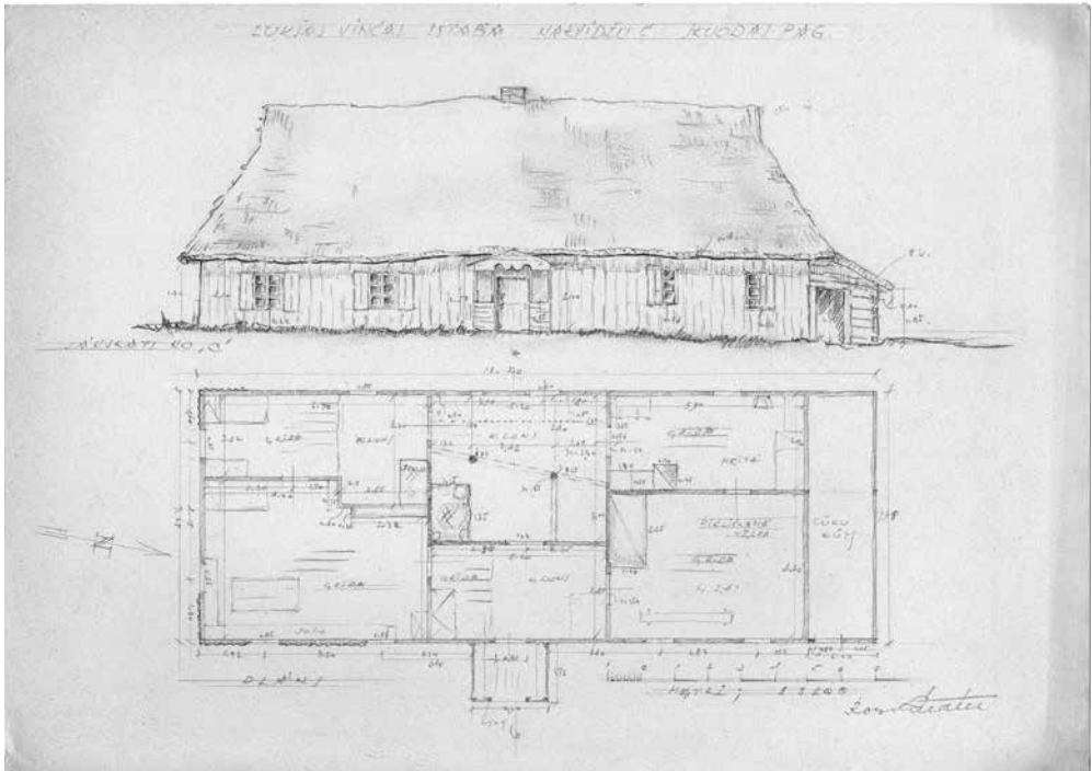
Narvydžių km. V. Lukšo sodybos troba (virš durų yra skaičius 1768), su prieangiu, kaminu, pušis, eglė. 1942 m. LNVN, ZAE, Lietuva, segt. 4, ank. 1329. R. Priedėtes pieš.
