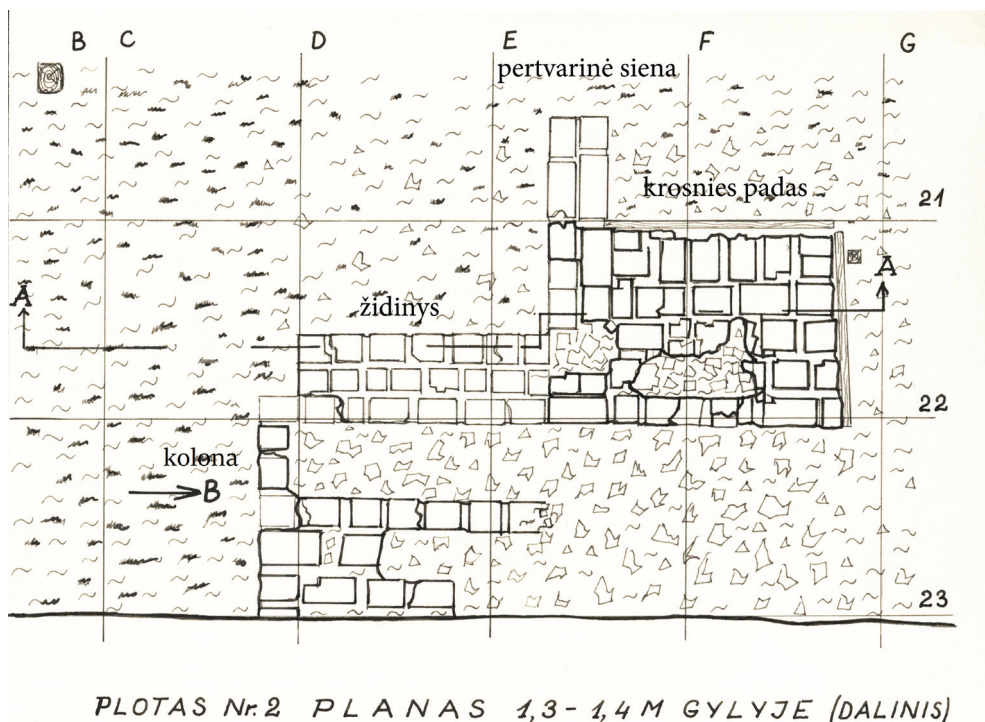
1 pav. Krosnies padas ir židinio vieta XVII a. fachverkinio namo viduje. Šaltinis: ŽULKUS, V. Gyvenamasis namas..., brėž. nr. 4 (autorė L. Žulkienė); MLIM, AS 38 (priešai R. Nabažaitės)
