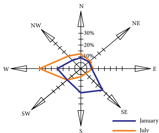
Fig. 5. Wind-rose
