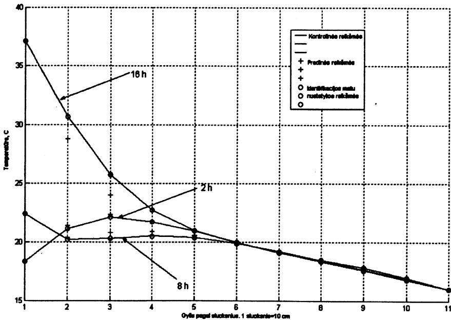
1 pav. Dirvožemio temperatūros profilai.
